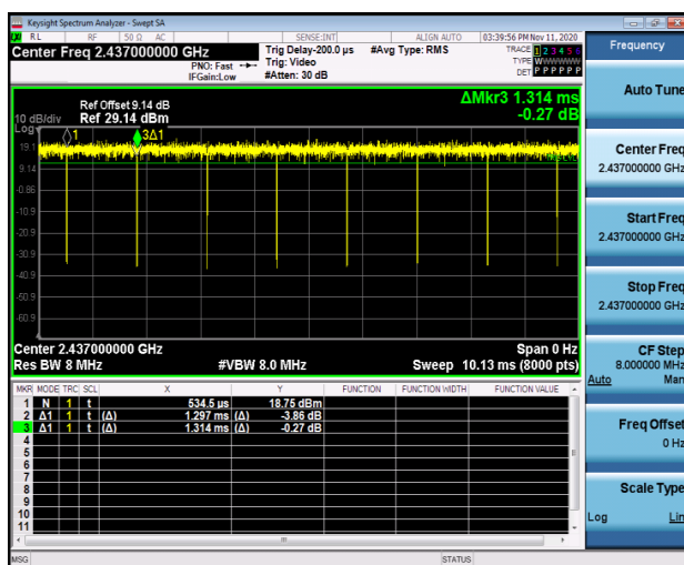
802.11n HT20
