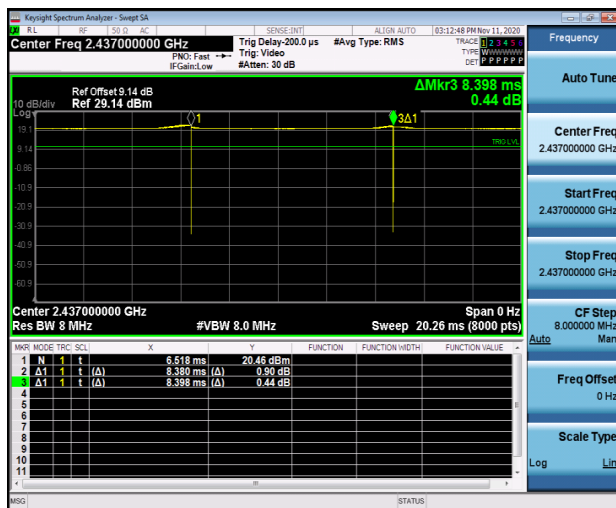
802.11b
