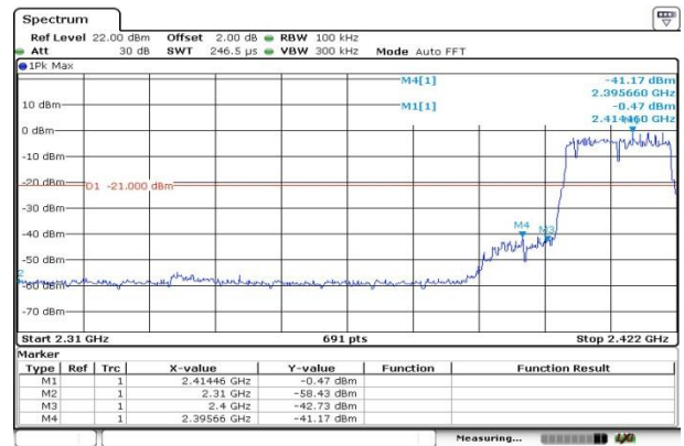
CH01-Bandedge
