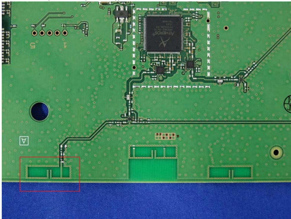
(17) EUT Photo (Antenna: (ANT1A))
