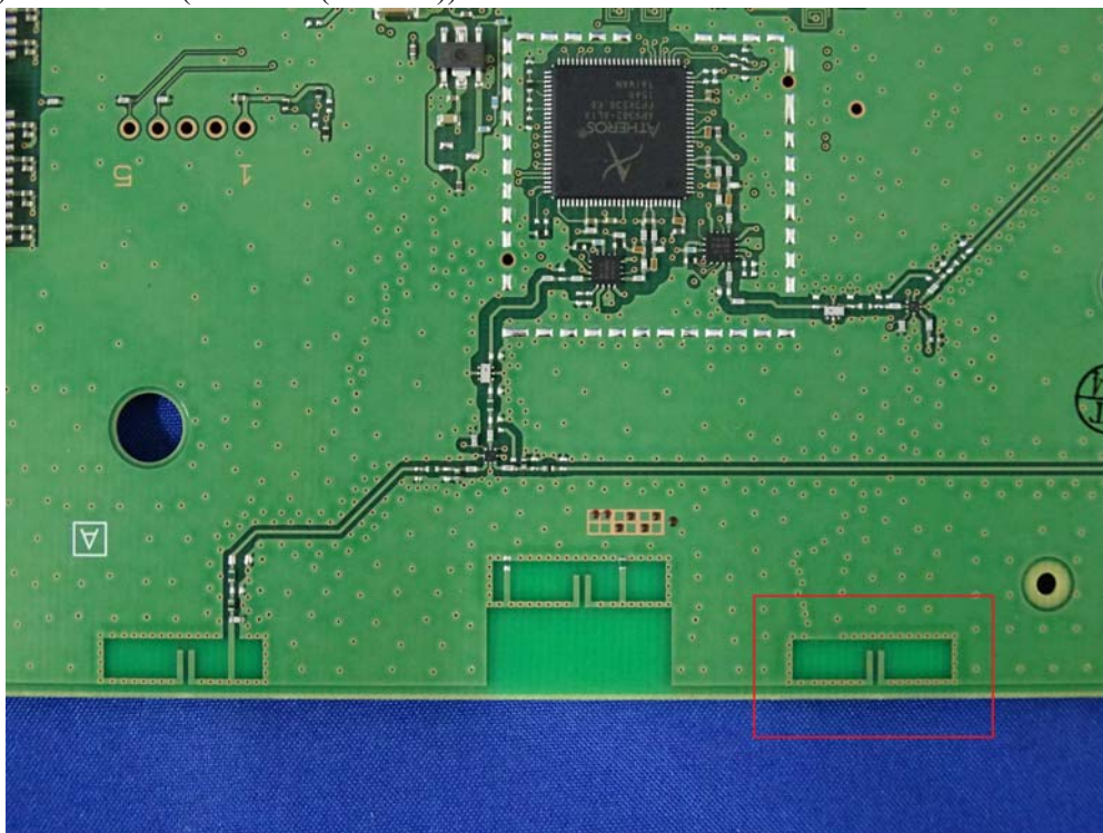
(18) EUT Photo (Antenna: (ANT0A))
