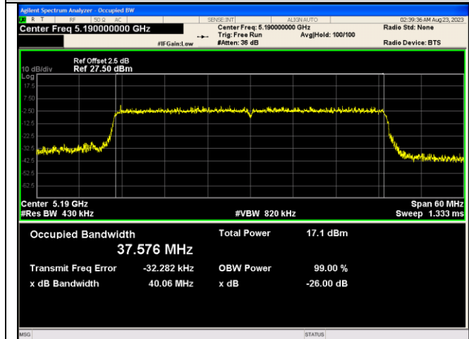
IEEE 802.11ax_Channel 38_40MHz_Antenna 0_RU&amp;Index 484RU65
