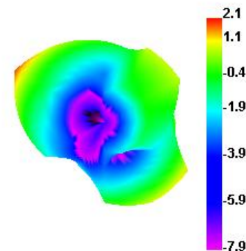
2450.000MHz
