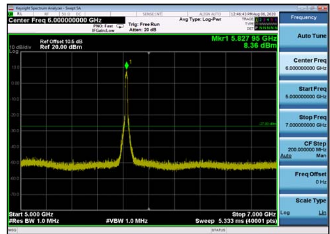
U-NII-3 ,Plot 3,5000MHz~7000MHz-802.1 1ac(20MHz),5825MHz,Ant1
