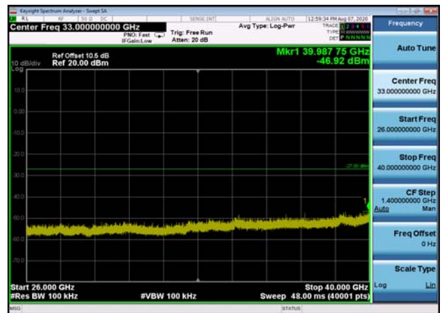
U-NII-3 ,Plot 2,26000MHz~40000MHz-802 .11ac(20MHz),5785MHz,Ant1
