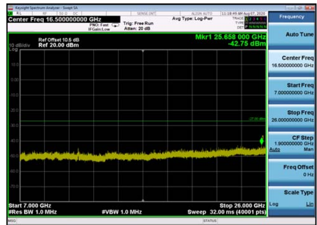
U-NII-3 ,Plot 4,7000MHz~26000MHz-802. 11ac(80MHz),5775MHz,Ant1
