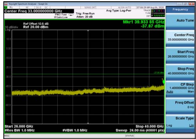
U-NII-1 ,Plot 2,26000MHz~40000MHz-802 .11ac(80MHz),5210MHz,Ant1
