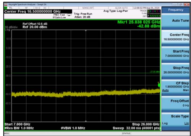
U-NII-3 ,Plot 4,7000MHz~26000MHz-802. 11n(20MHz),5825MHz,Ant1
