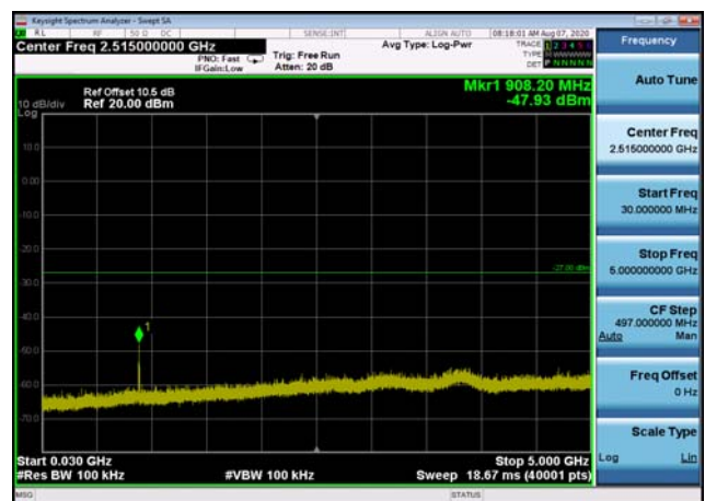
U-NII-3 ,Plot 2,30MHz~5000MHz-802.11n (40MHz),5795MHz,Ant1
