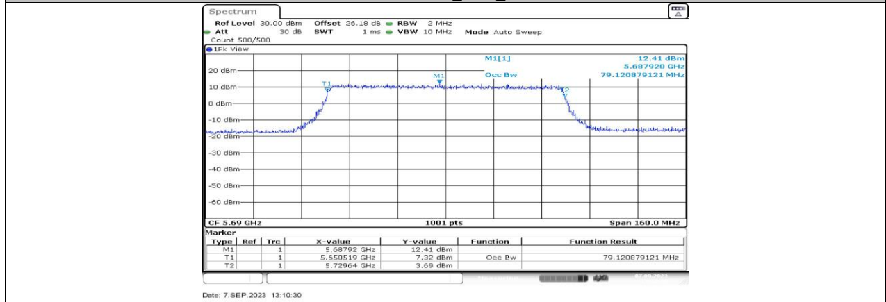
11BE80MIMO_Ant2_5690
