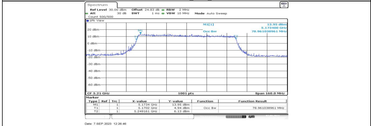
11BE80MIMO_Ant4_5210
