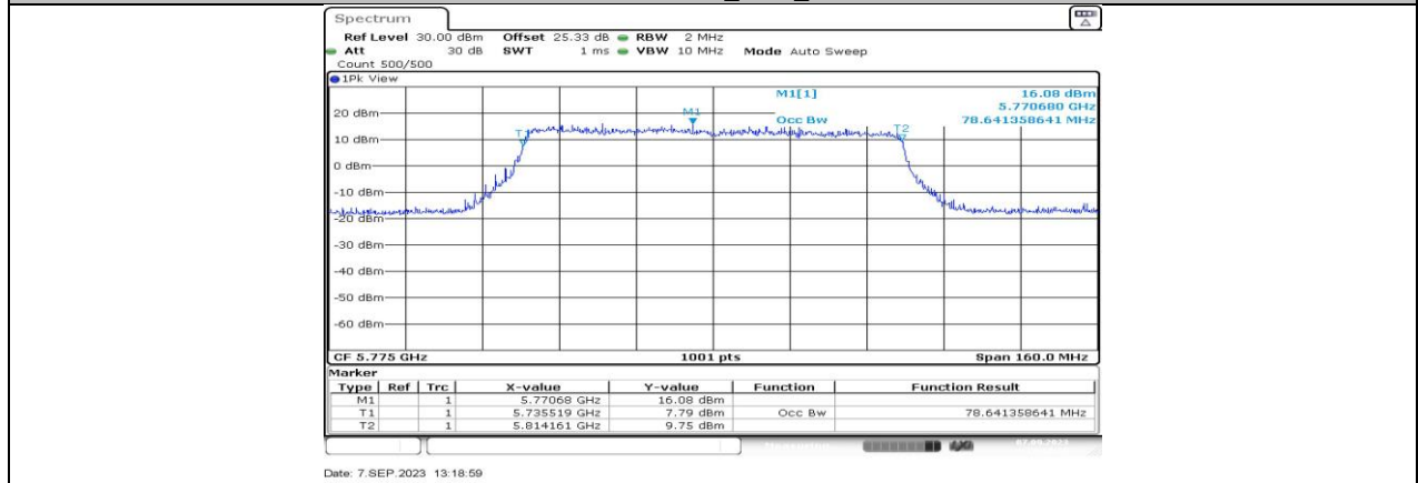
11BE80MIMO_Ant4_5775
