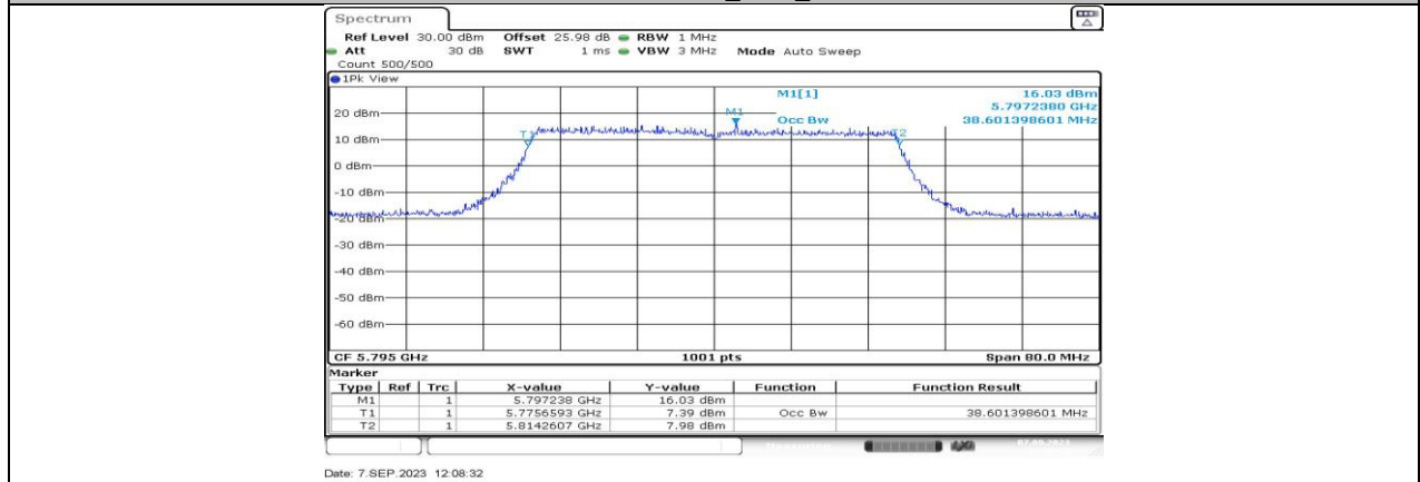
11BE40MIMO_Ant1_5795
