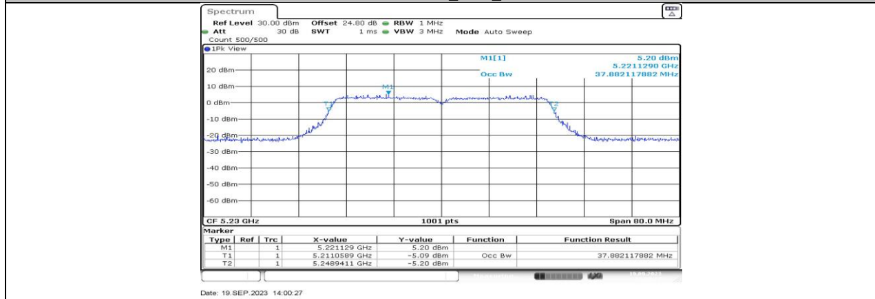
11AC40MIMO_Ant3_5230
