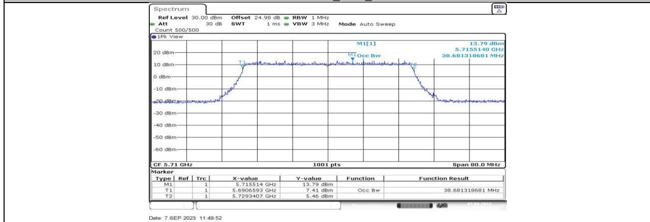
11BE40MIMO_Ant2_5710
