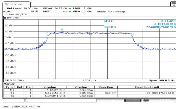
11AC80MIMO_Ant4_5210
