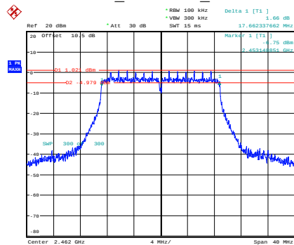
n20_2462MHz_Chain 0
