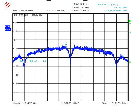
b_2437MHz_Chain 0
