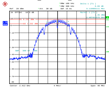
b_2412MHz_Chain 0
