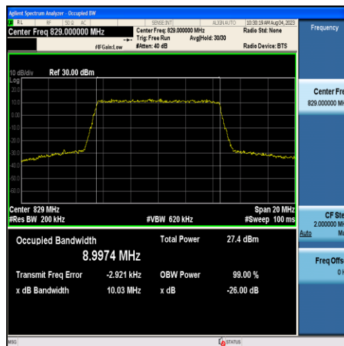
Band26-10MHz-QPSK-26840-50RB#0-8.9974
