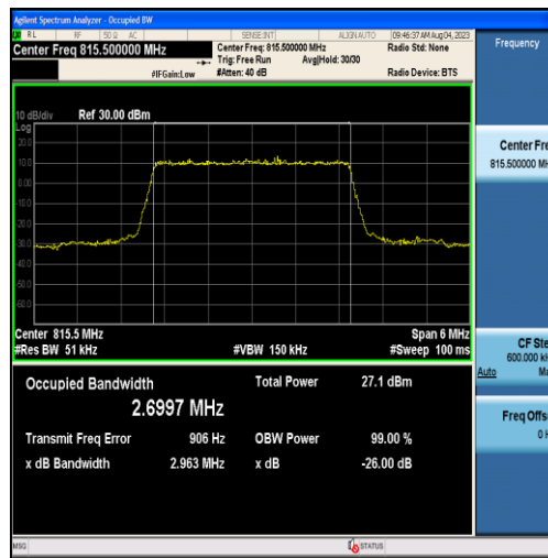
Band26-3MHz-QPSK-26705-15RB#0-2.6997
