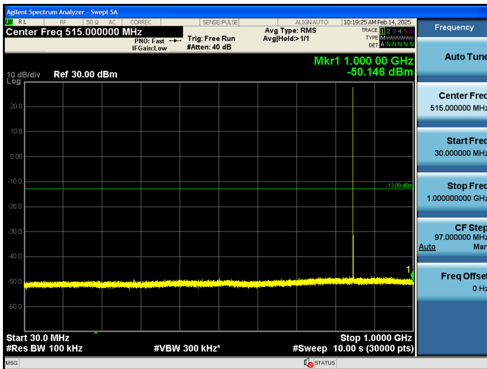
Test_Graph_bandGSM850_848.8MHz_GPRS 1Slot_30M_1G_TX
