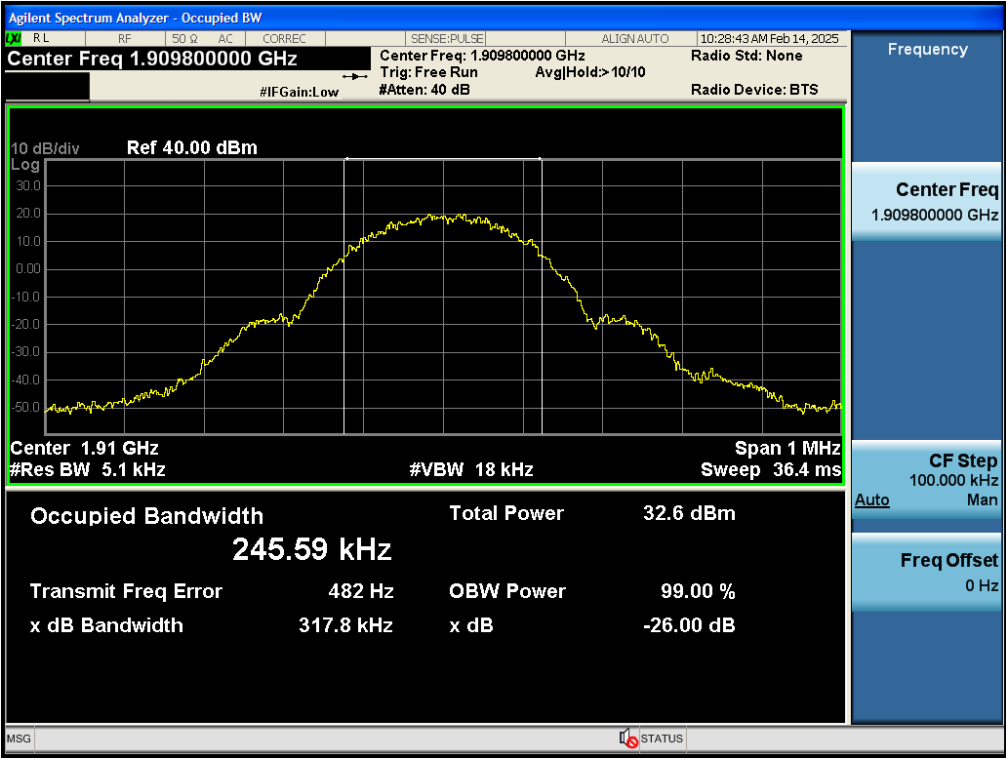
Test_Graph_bandGSM1900_1909.8MHz_GPRS 1Slot_OBW&EBW
