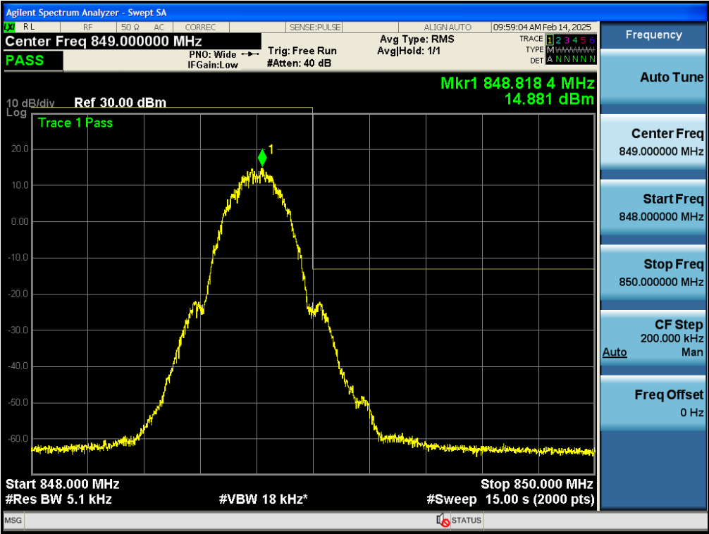
Test_Graph_bandGSM850_848.8MHz_GPRS 1Slot_Band edge
