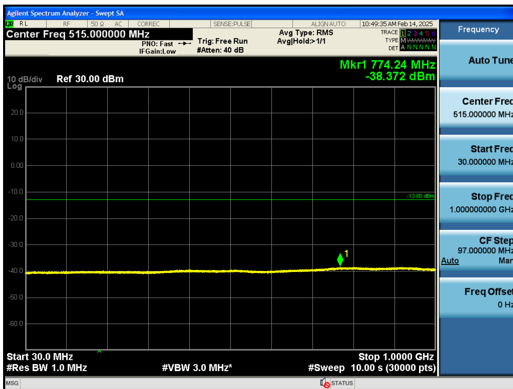
Test_Graph_bandGSM1900_1909.8MHz_GPRS 1Slot_30M_1G_TX
