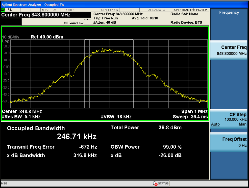
Test_Graph_bandGSM850_848.8MHz_Voice_OBW&EBW
