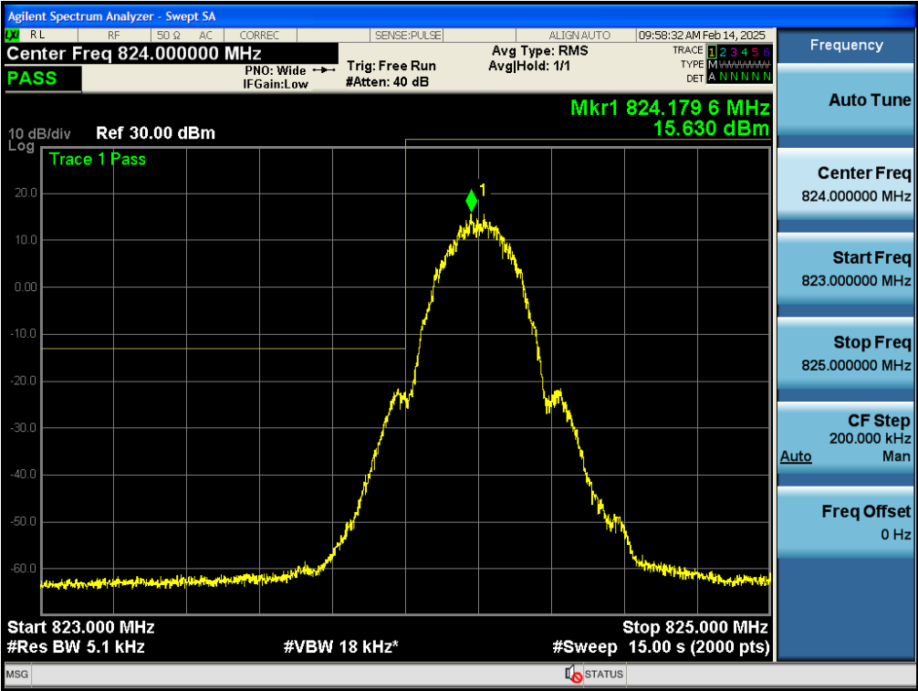
Test_Graph_bandGSM850_824.2MHz_GPRS 1Slot_Band edge
