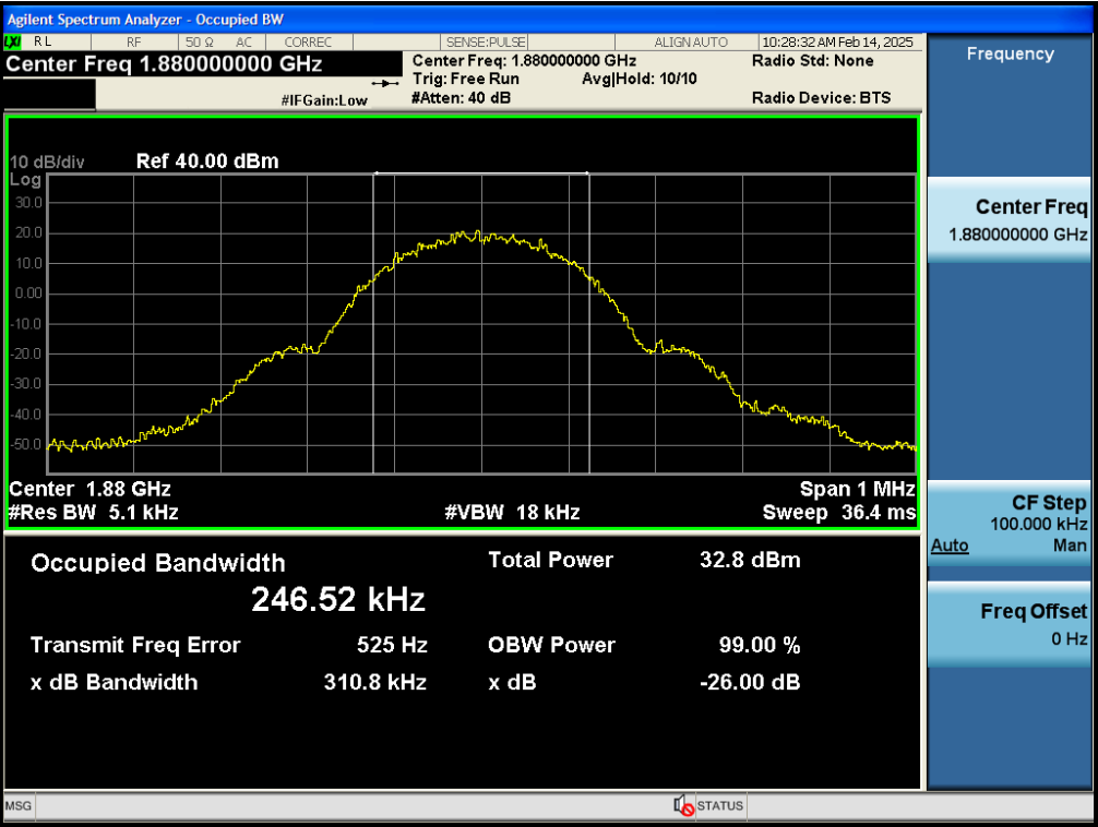
Test_Graph_bandGSM1900_1880MHz_GPRS 1Slot_OBW&EBW
