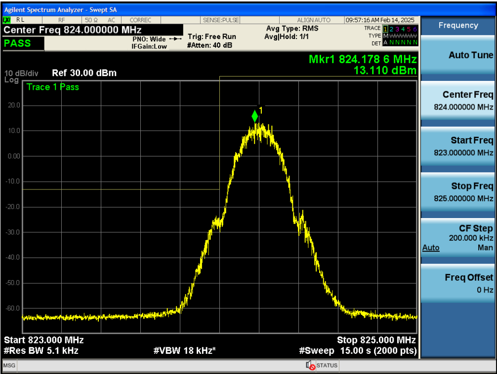
Test_Graph_bandGSM850_824.2MHz_Voice_Band edge
