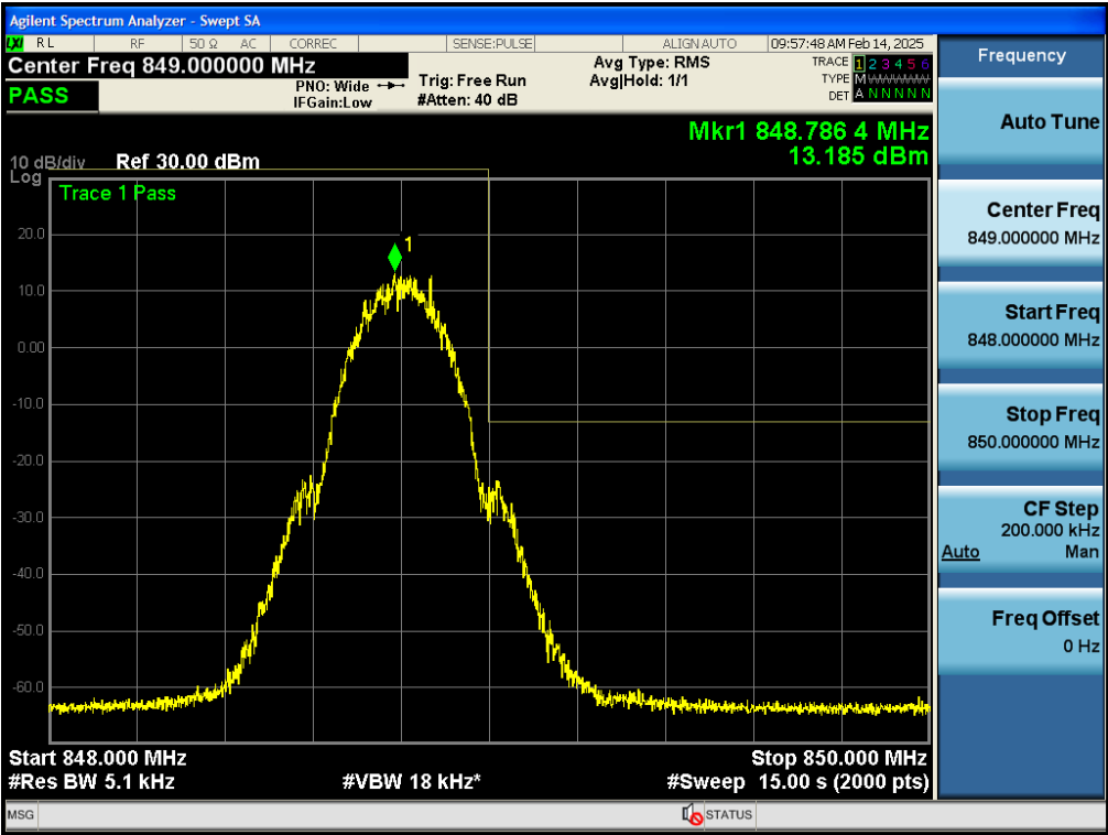
Test_Graph_bandGSM850_848.8MHz_Voice_Band edge
