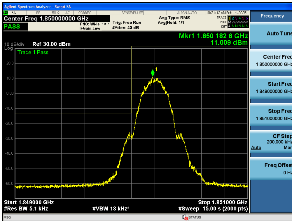
Test_Graph_bandGSM1900_1850.2MHz_GPRS 1Slot_Band edge
