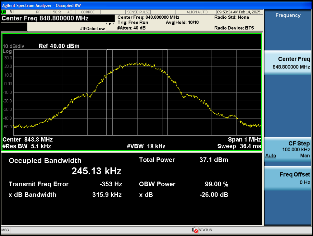
Test_Graph_bandGSM850_848.8MHz_GPRS 1Slot_OBW&EBW
