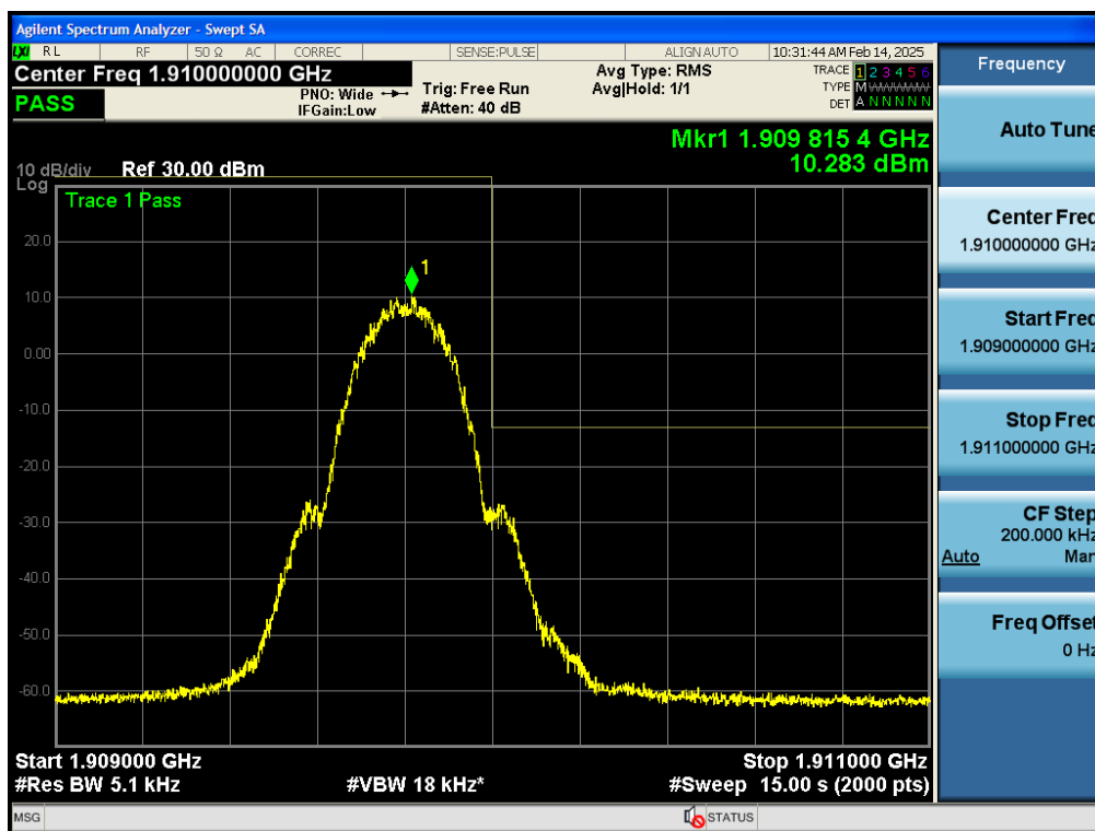
Test_Graph_bandGSM1900_1909.8MHz_GPRS 1Slot_Band edge
