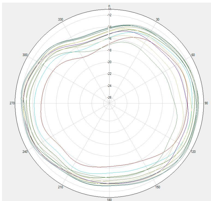
LTE B12/B13/B17/B28 Theta=90deg
