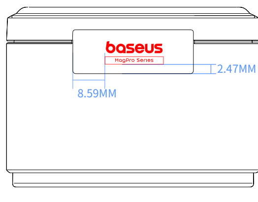
前视图
