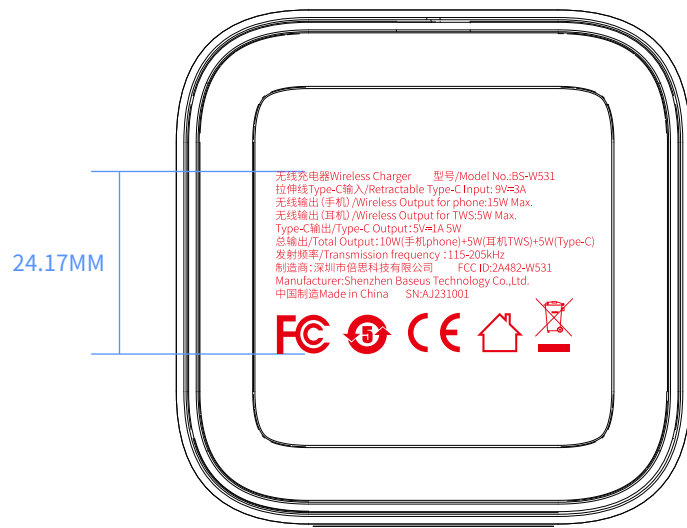
底视图
