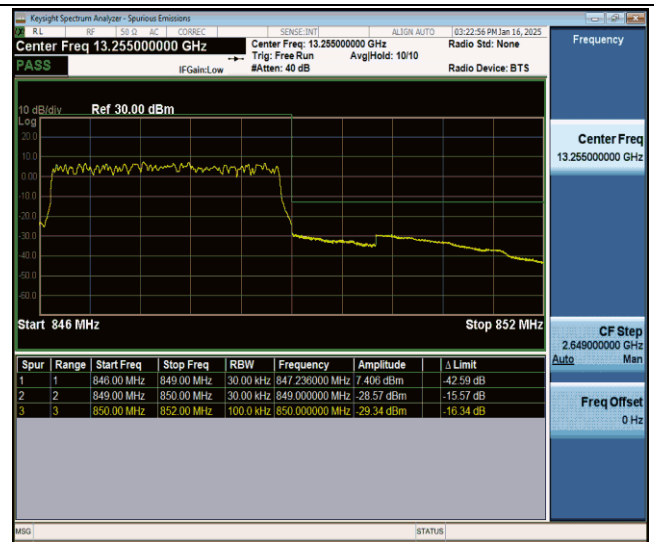
Band26(824-849)-3MHz-QPSK-27025-15RB#0-PASS
