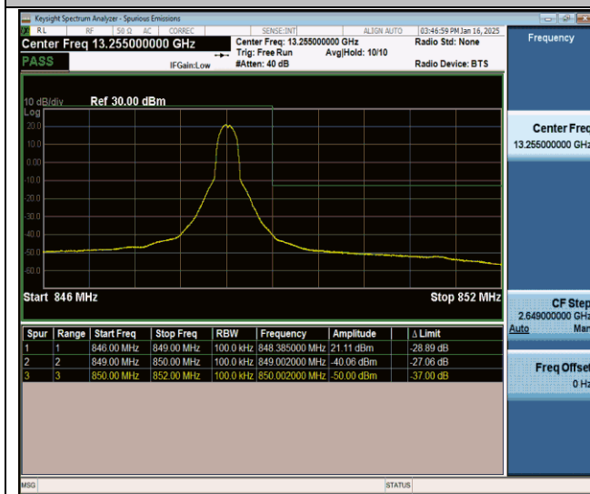
Band26(824-849)-10MHz-QPSK-26990-1RB#49-PASS
