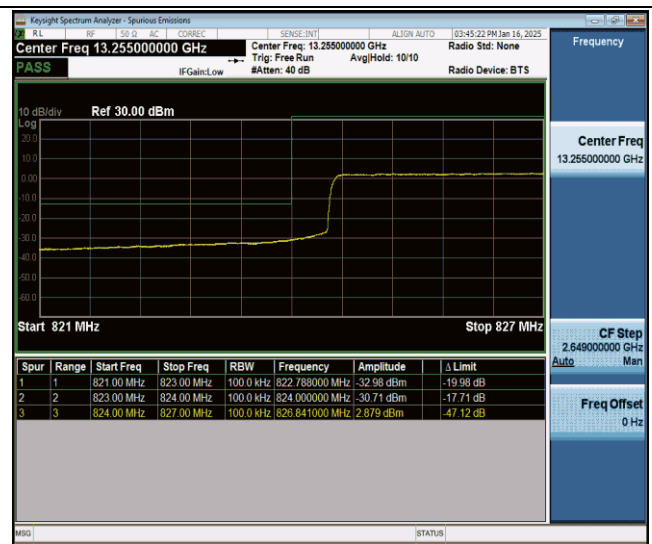
Band26(824-849)-10MHz-QPSK-26840-50RB#0-PASS
