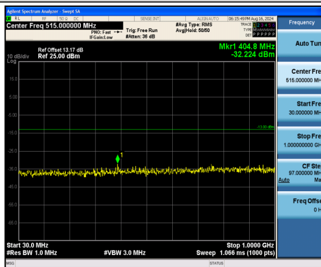
Band2-20MHz-QPSK-19100-1RB#0-Range4:1000~2000MHz
