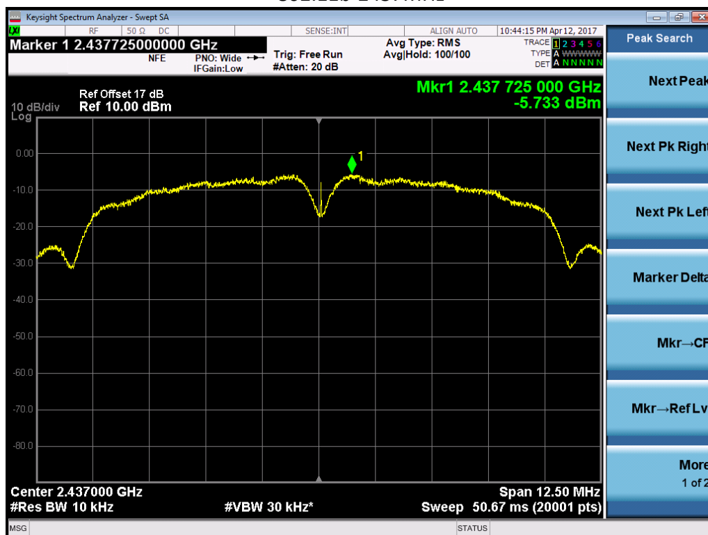
802.11b-2437MHz
