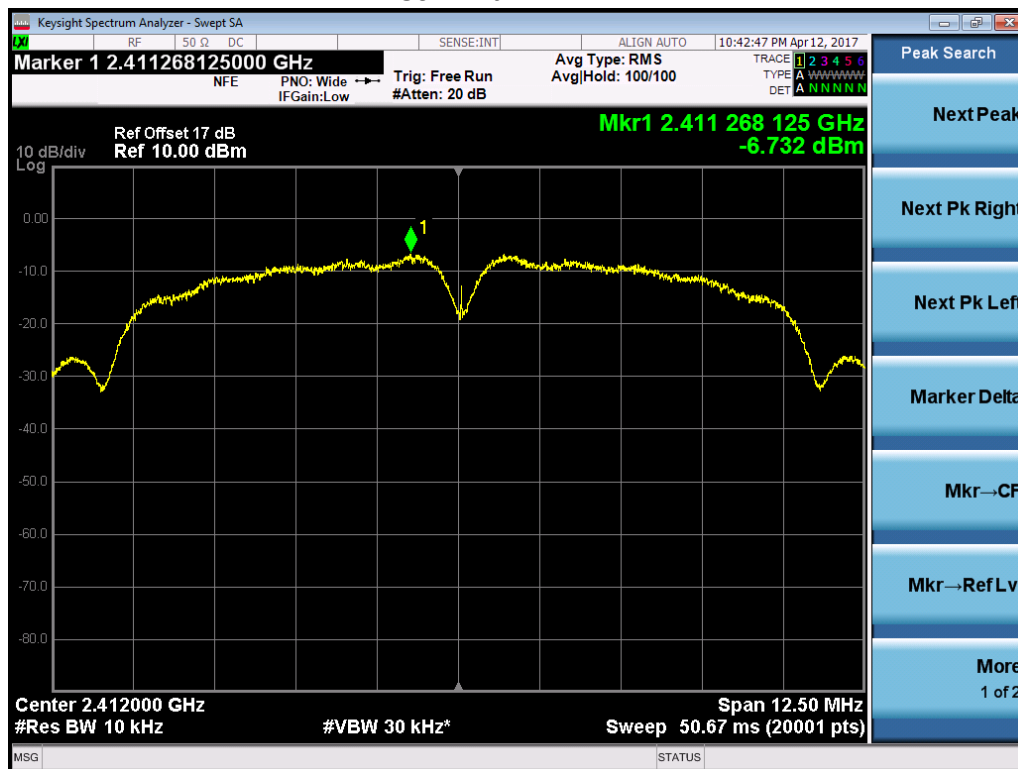
802.11b-2412MHz
