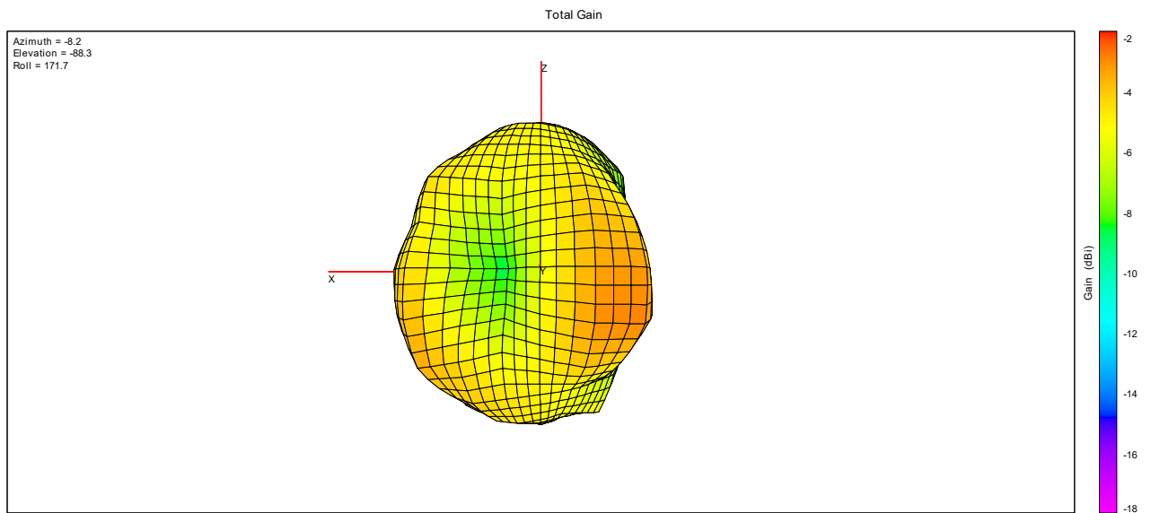
2480MHz_2#_MS-661
