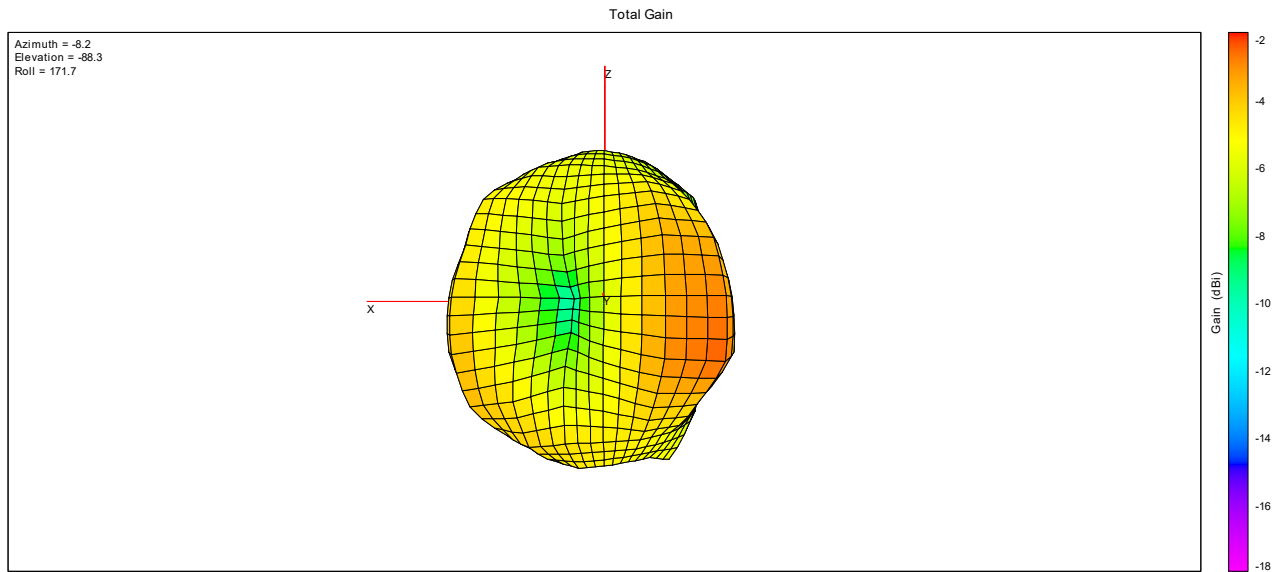
2440MHz_2#_MS-661
