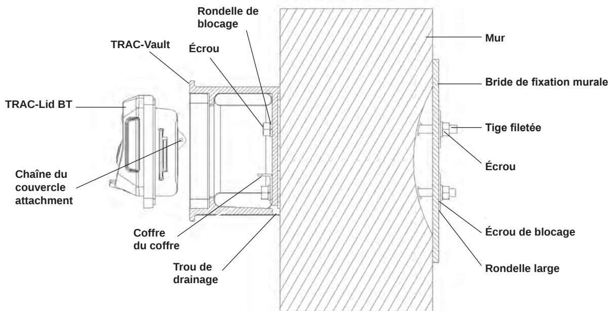
Image 5. TRAC-Vault BT installé dans le mur, vue latérale
