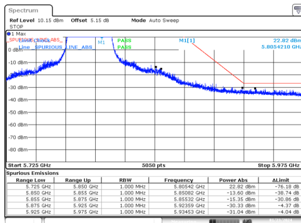
BE-NR-HIGH, MIMO-A, 802.11n40-HT0, Ch159
