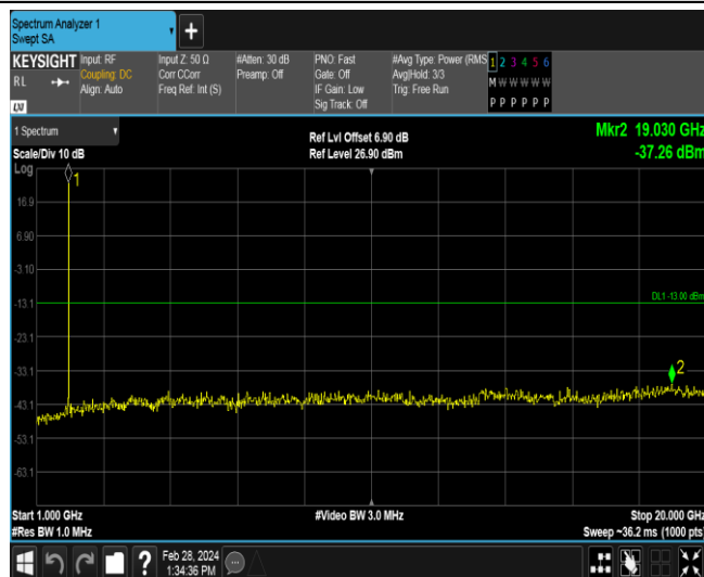
Band2-3MHz-QPSK-19185-1RB#0-Range2:1000~20000MHz
