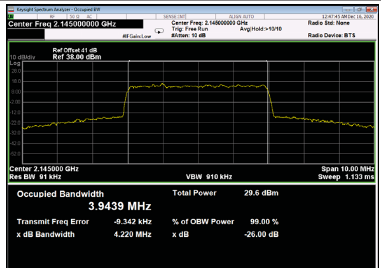
Figure 672: 256QAM 5MHz B.W.; 2145.0MHz, 30kHz - Output
