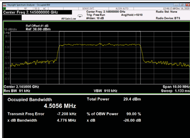
Figure 671: 256QAM 5MHz B.W.; 2145.0MHz, 15kHz - Output
