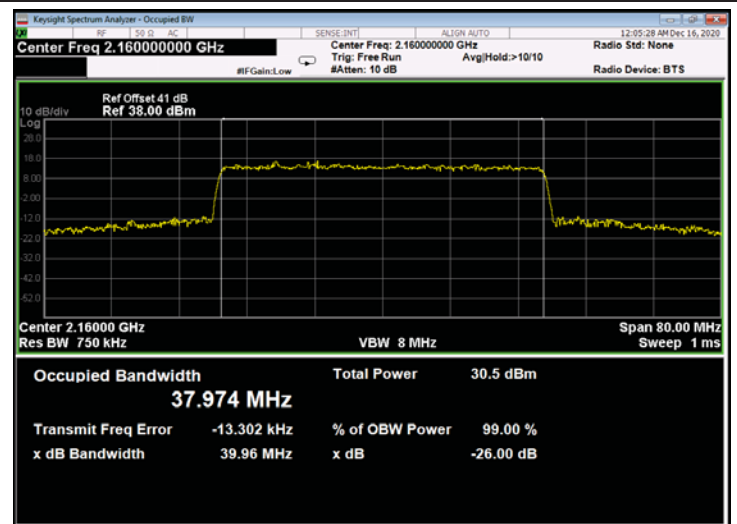
Figure 652: 64QAM 40MHz B.W.; 2160.0MHz, 30kHz - Output
