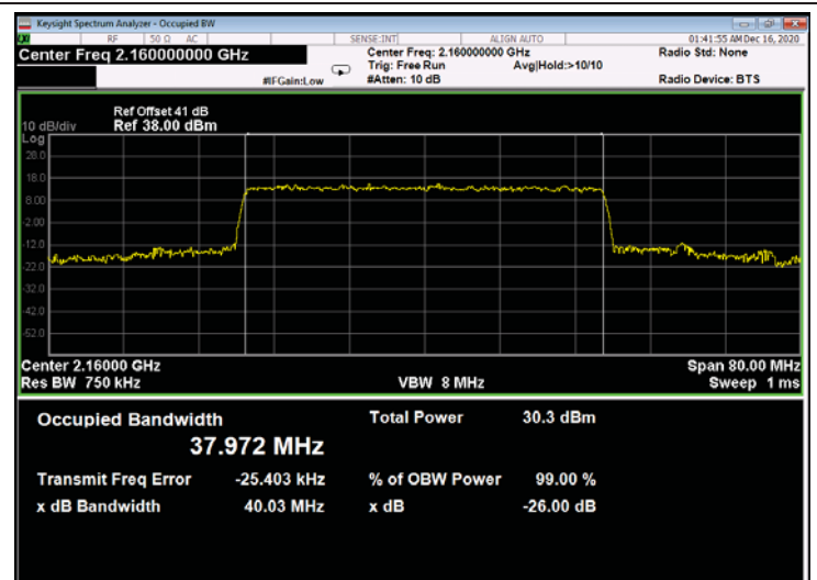
Figure 718: 256QAM 40MHz B.W.; 2160.0MHz, 30kHz - Output
