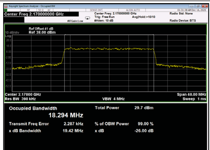
Figure 700: 256QAM 20MHz B.W.; 2170.0MHz, 30kHz - Output
