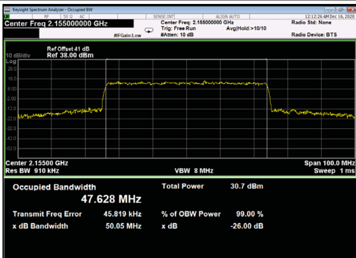
Figure 661: 64QAM 50MHz B.W.; 2155.0MHz, 30kHz - Output
