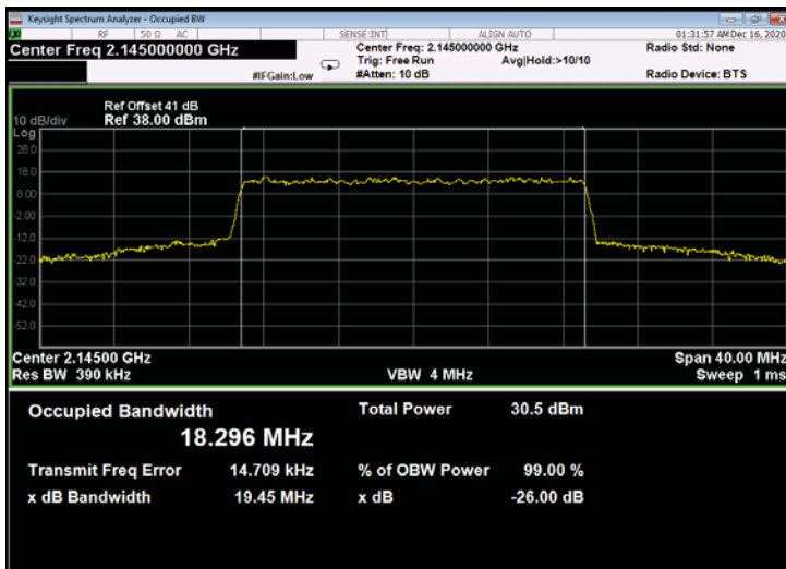
Figure 697: 256QAM 20MHz B.W.; 2145.0MHz, 30kHz - Output
