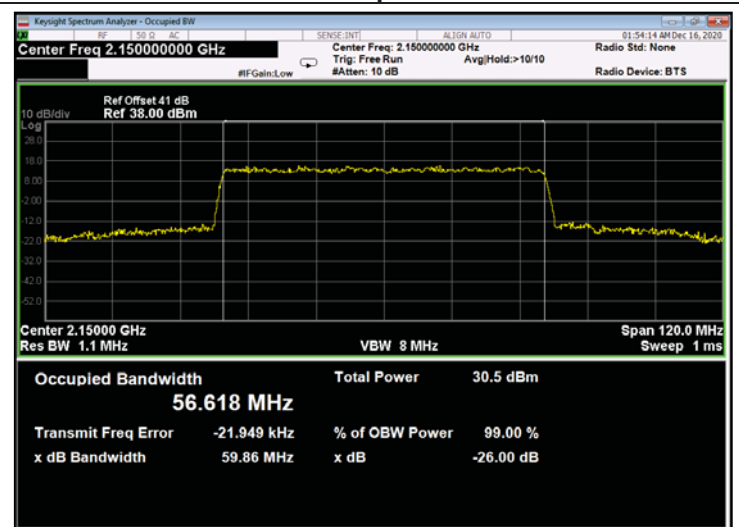
Figure 734: 256QAM 60MHz B.W.; 2150.0MHz, 60kHz - Output
