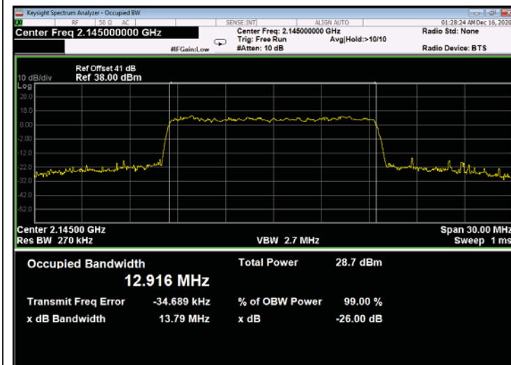
Figure 689: 256QAM 15MHz B.W.; 2145.0MHz, 60kHz - Output
