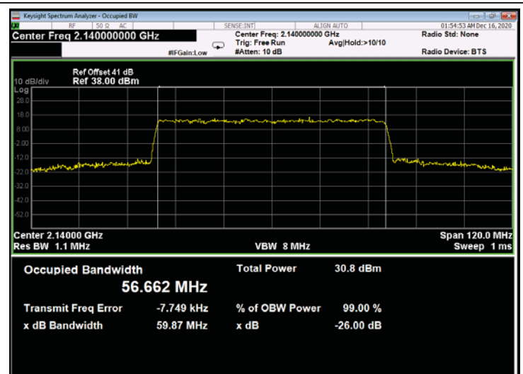
Figure 730: 256QAM 60MHz B.W.; 2140.0MHz, 60kHz - Output
