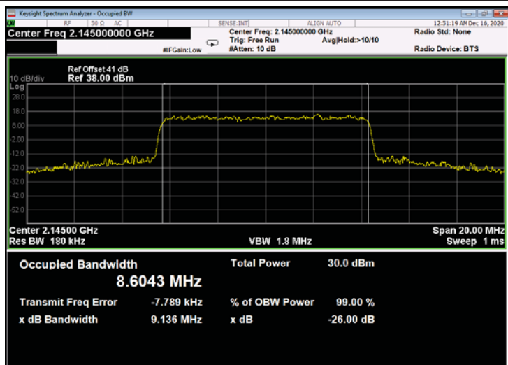
Figure 679: 256QAM 10MHz B.W.; 2145.0MHz, 30kHz - Output
