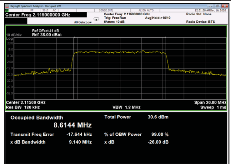
Figure 676: 256QAM 10MHz B.W.; 2115.0MHz, 30kHz - Output
