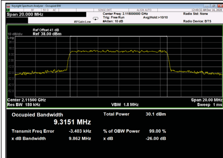
Figure 675: 256QAM 10MHz B.W.; 2115.00MHz, 15kHz - Output
