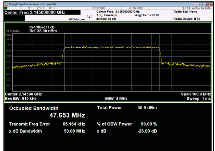
Figure 658: 64QAM 50MHz B.W.; 2145MHz, 30kHz - Output
