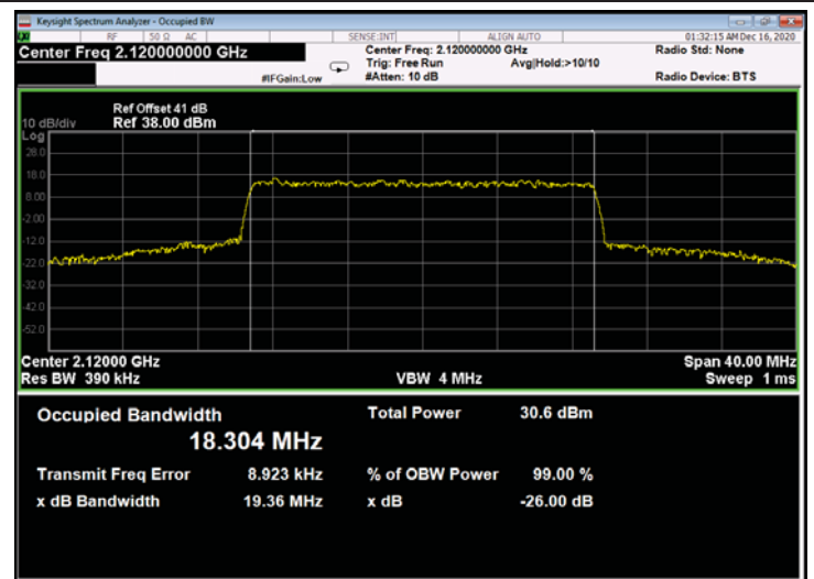
Figure 694: 256QAM 20MHz B.W.; 2120.0MHz, 30kHz - Output
