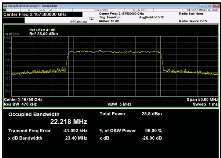
Figure 710: 256QAM 25MHz B.W.; 2167.5MHz, 60kHz - Output
