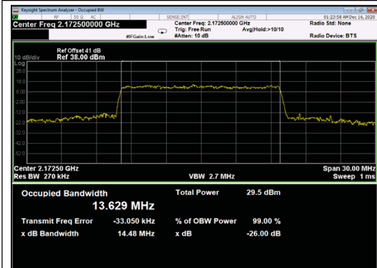
Figure 691: 256QAM 15MHz B.W.; 2172.5MHz, 30kHz - Output
