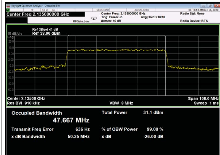
Figure 721: 256QAM 50MHz B.W.; 2135.0MHz, 30kHz - Output
