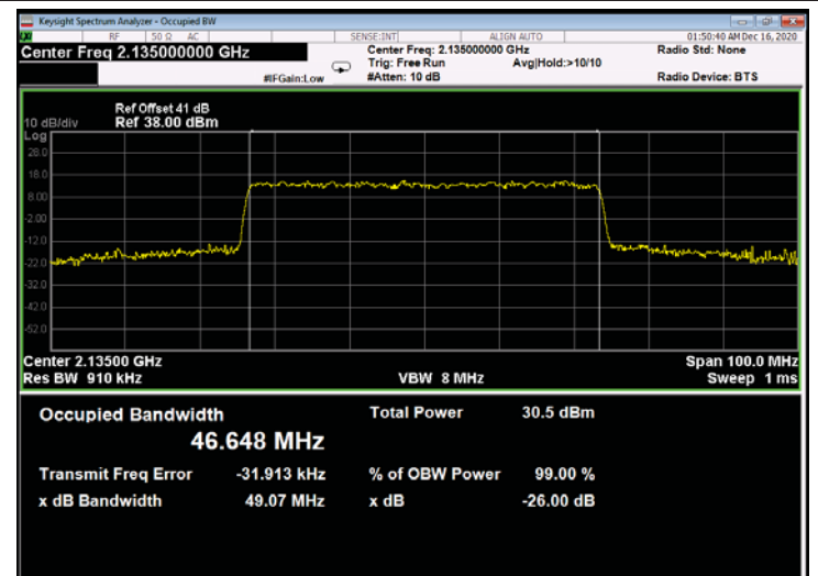
Figure 722: 64QAM 50MHz B.W.; 2135.0MHz, 60kHz - Output
