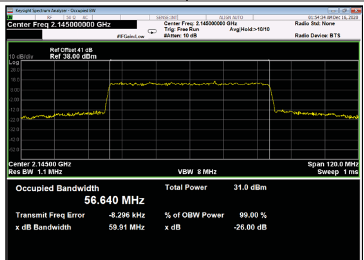
Figure 732: 256QAM 60MHz B.W.; 2145.0MHz, 60kHz - Output
