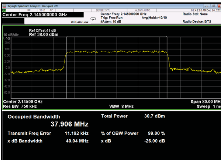
Figure 715: 256QAM 40MHz B.W.; 2145.0MHz, 30kHz - Output
