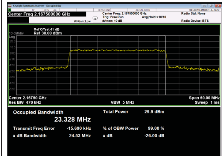
Figure 709: 256QAM 25MHz B.W.; 2167.5MHz, 30kHz - Output
