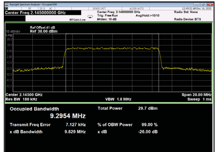
Figure 678: 256QAM 10MHz B.W.; 2145.0MHz, 15kHz - Output
