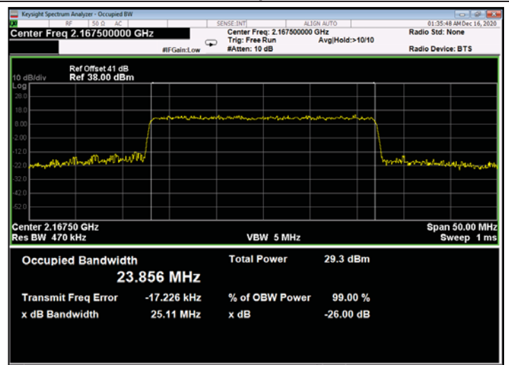
Figure 708: 256QAM 25MHz B.W.; 2167.5MHz, 15kHz - Output
