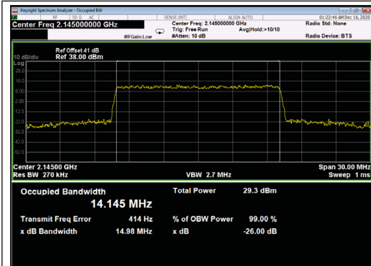
Figure 687: 256QAM 15MHz B.W.; 2145.0MHz, 15kHz - Output
