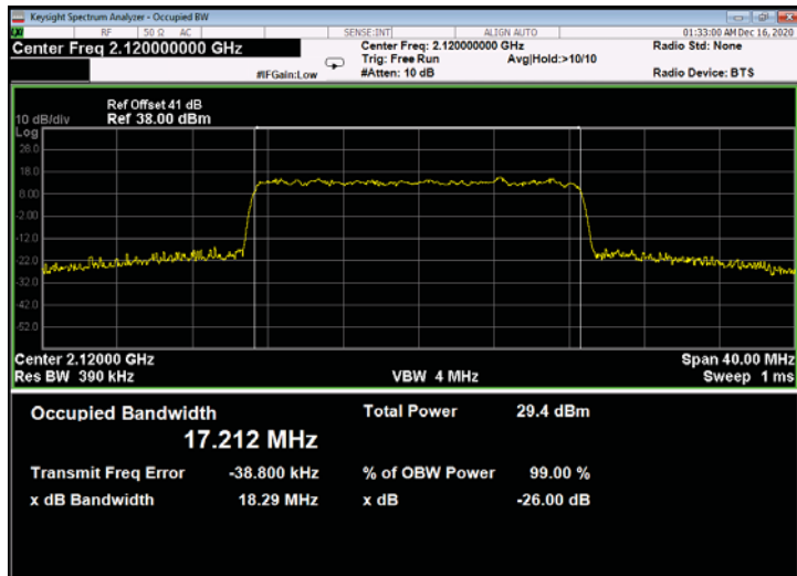
Figure 695: 256QAM 20MHz B.W.; 2120.0MHz, 60kHz - Output
