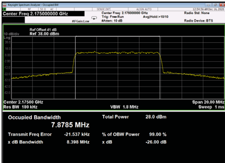
Figure 683: 256QAM 10MHz B.W.; 2175.0MHz, 60kHz - Output
