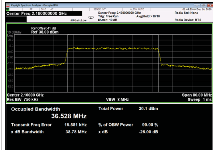
Figure 719: 256QAM 40MHz B.W.; 2160.0MHz, 60kHz - Output
