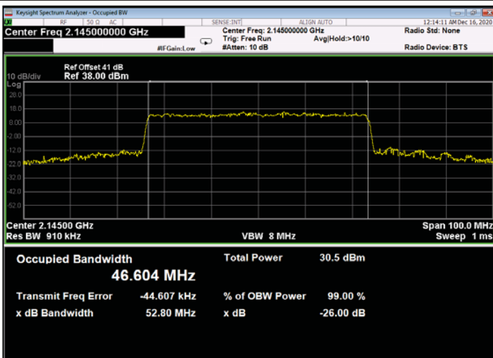
Figure 659: 64QAM 50MHz B.W.; 2145MHz, 60kHz - Output
