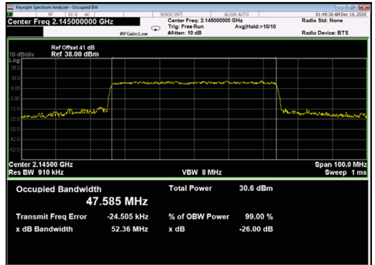
Figure 724: 256QAM 50MHz B.W.; 2145.0MHz, 30kHz - Output
