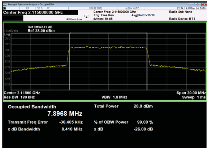
Figure 677: 256QAM 10MHz B.W.; 2115.0MHz, 60kHz - Output
