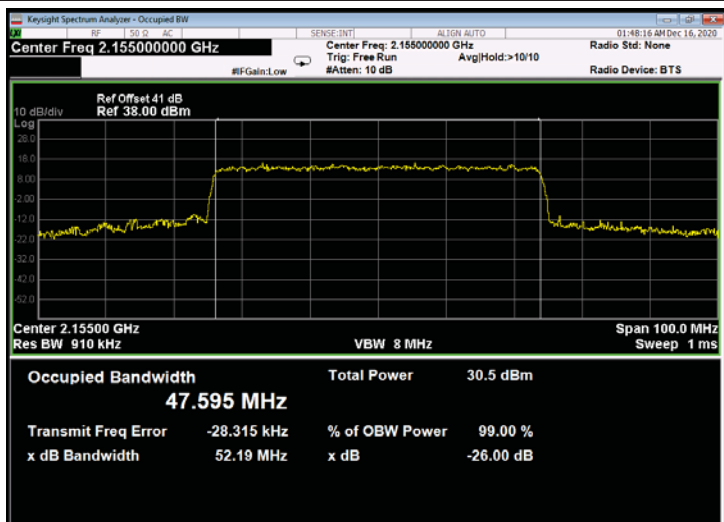
Figure 727: 256QAM 50MHz B.W.; 2155.0MHz, 30kHz - Output
