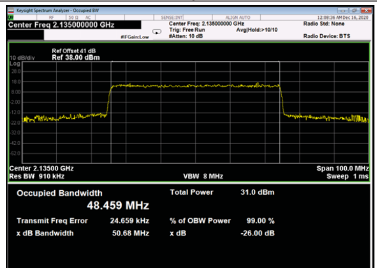
Figure 654: 64QAM 50MHz B.W.; 2135.0MHz, 15kHz - Output
