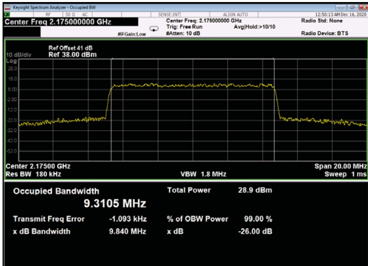
Figure 681: 256QAM 10MHz B.W.; 2175.0MHz, 15kHz - Output
