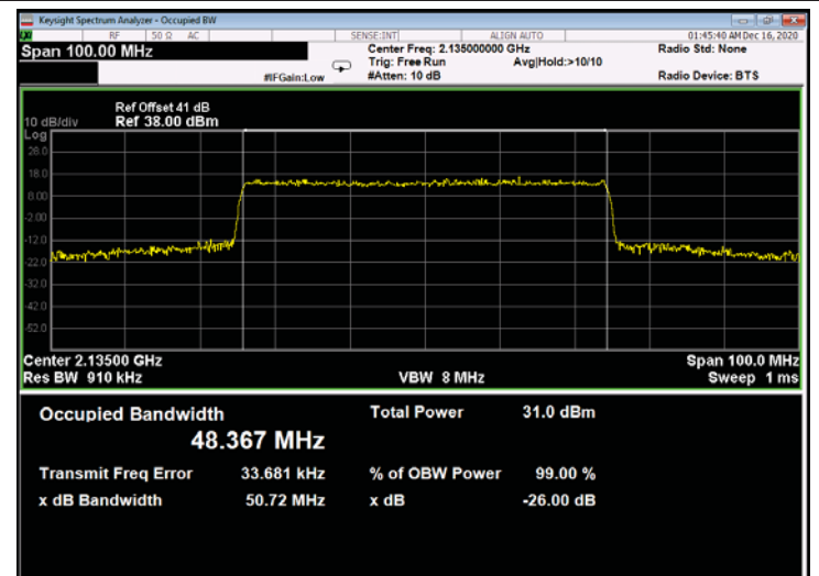
Figure 720: 256QAM 50MHz B.W.; 2135.0MHz, 15kHz - Output
