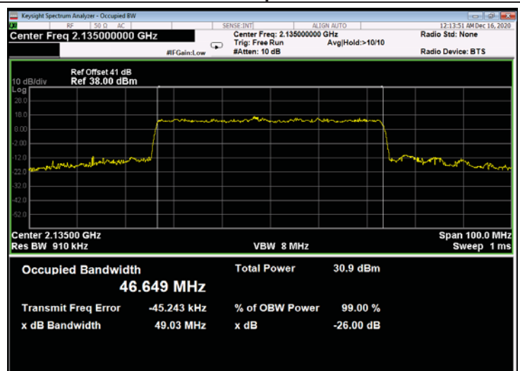
Figure 656: 64QAM 50MHz B.W.; 2135.0MHz, 60kHz - Output
