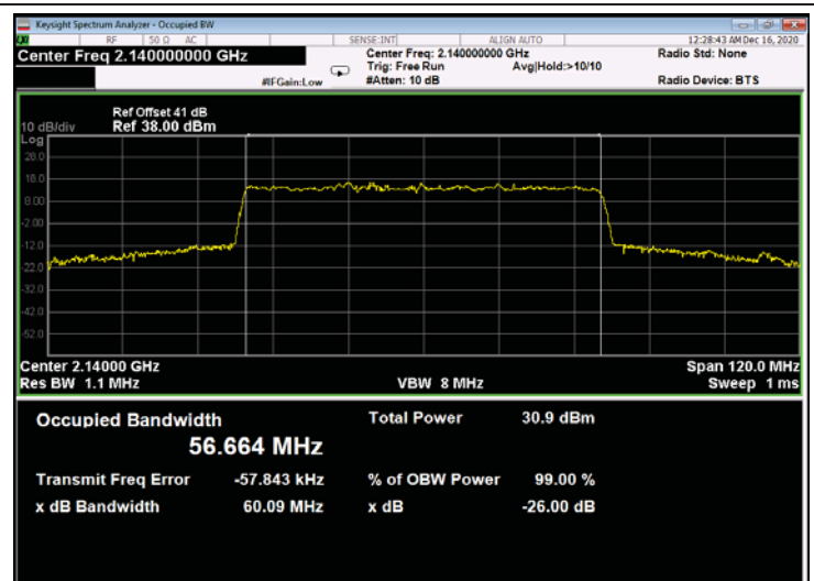
Figure 664: 64QAM 60MHz B.W.; 2140.0MHz, 60kHz - Output
