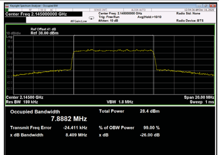
Figure 680: 256QAM 10MHz B.W.; 2145.0MHz, 60kHz - Output
