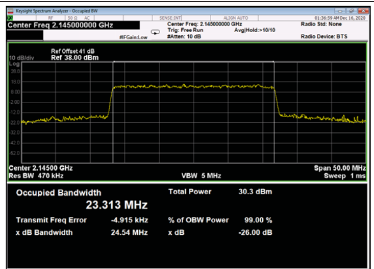
Figure 706: 256QAM 25MHz B.W.; 2145.0MHz, 30kHz - Output
