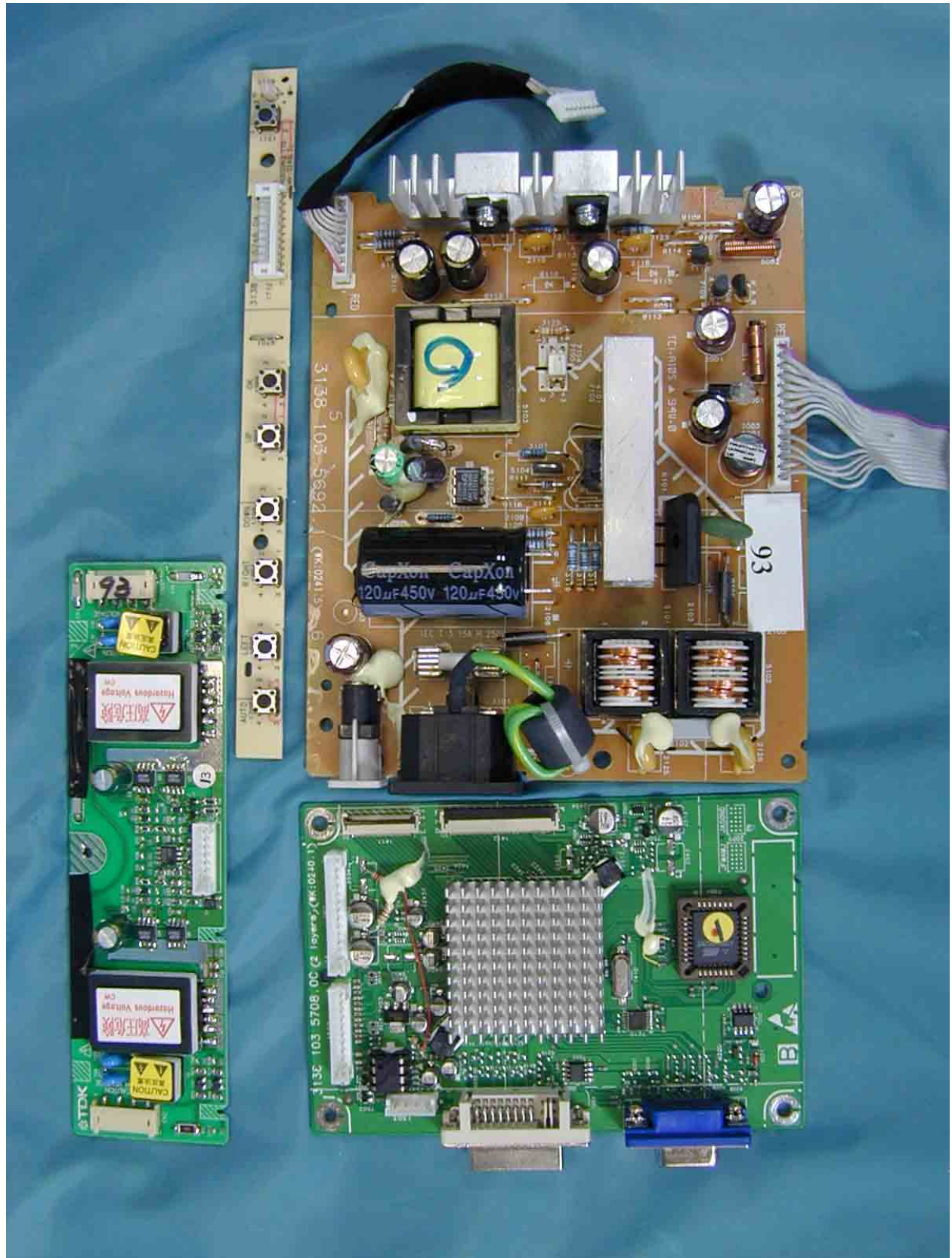
PCB Layout (AU Panel)
