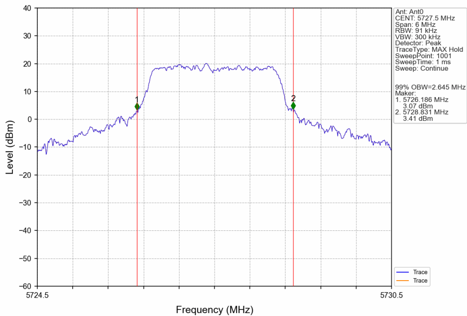
3M_LCH_5727.5MHz_Ant0_NTNV
