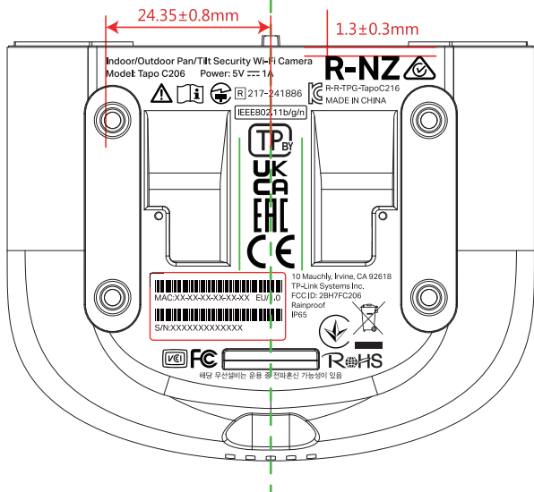
尺寸图
