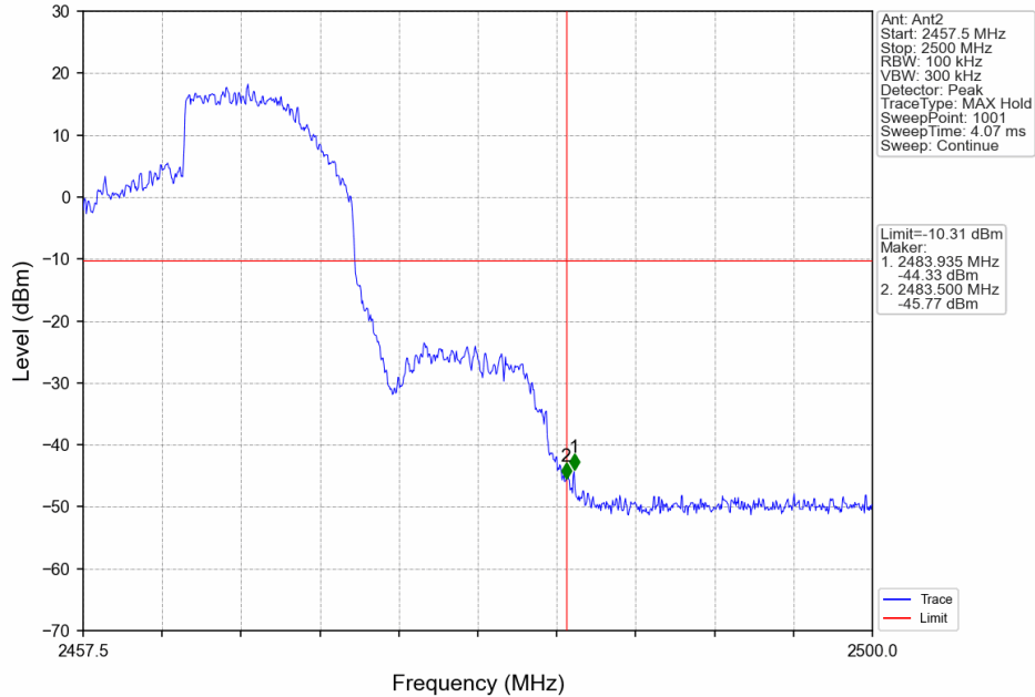
10M_HCH_2467.5MHz_Ant2_NTNV
