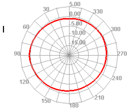
2441.000MHz H
