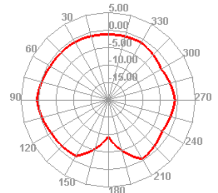
2441.000MHz E2
