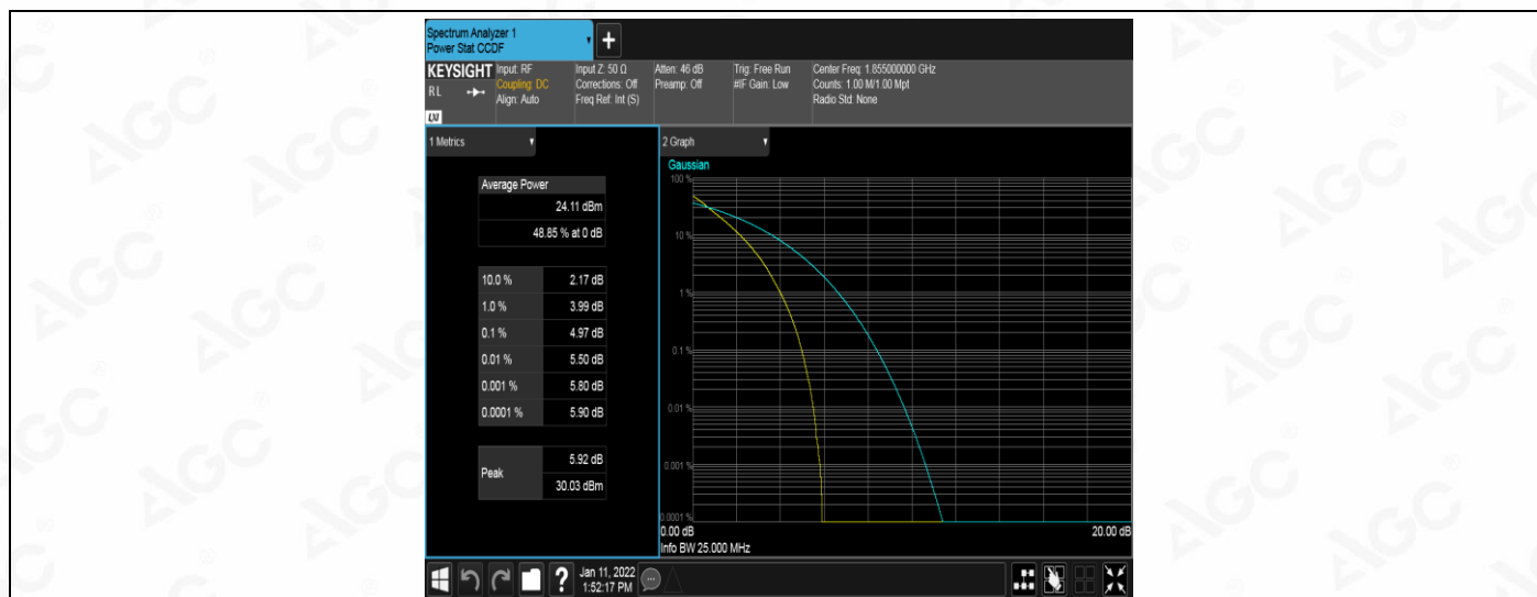
Band25-10MHz-QPSK-26365-1RB#0
