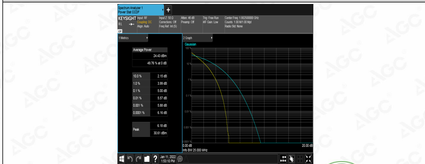
Band25-10MHz-QPSK-26365-50RB#0
