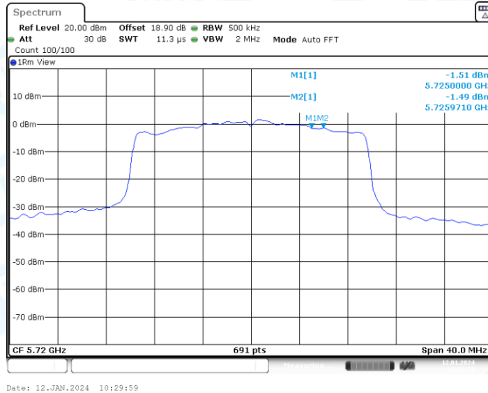
11AX20-CDD_Ant2_5720_UNII-3
