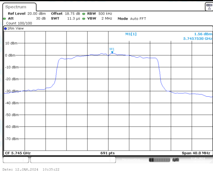
11AX20-CDD_Ant2_5745
