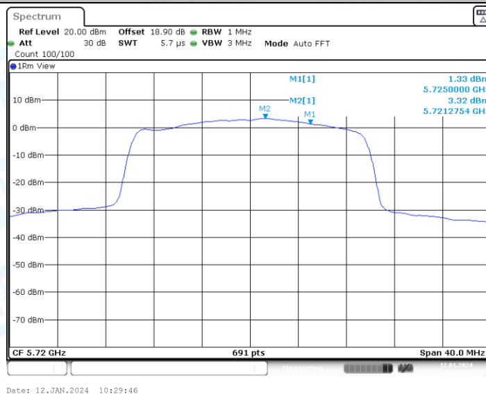
11AX20-CDD_Ant2_5720_UNII-2C
