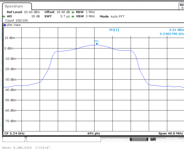
11AC20-CDD_Ant2_5240
