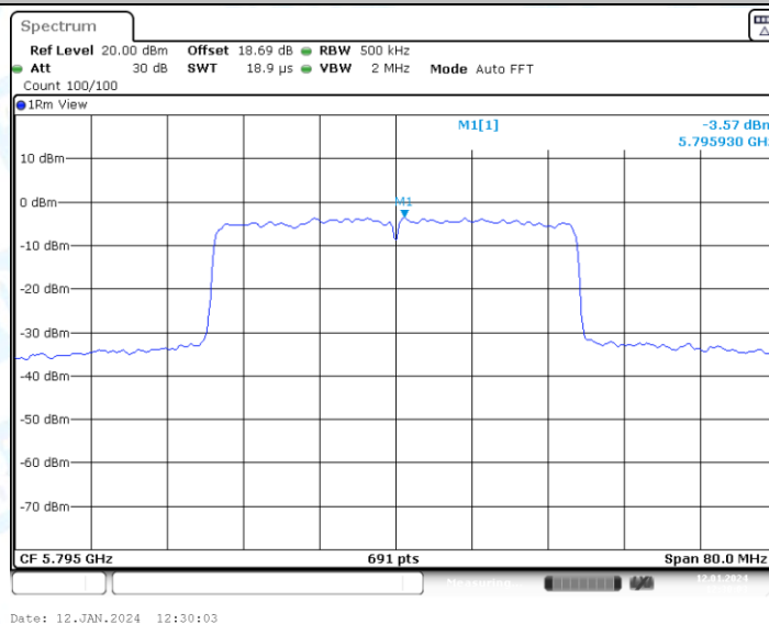
11AX40-CDD_Ant2_5795
