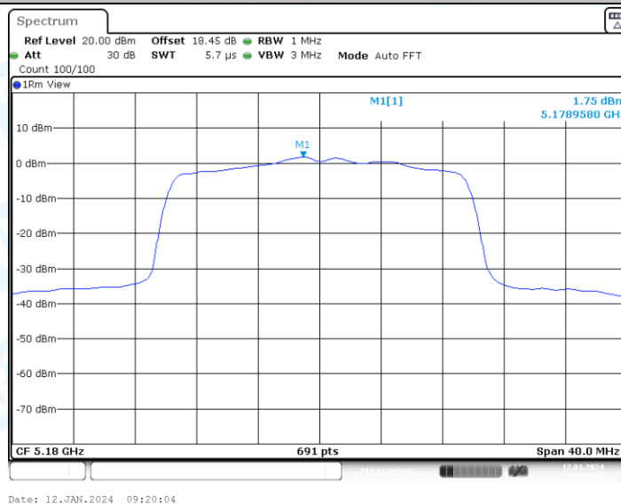
11AX20-CDD_Ant2_5180
