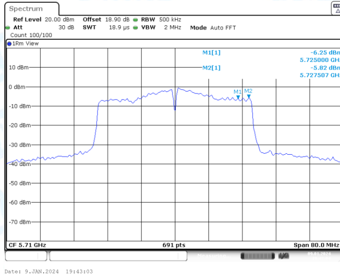
11AC40-CDD_Ant2_5710_UNII-3
