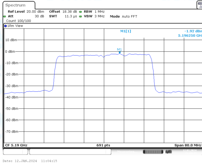
11AX40-CDD_Ant2_5190
