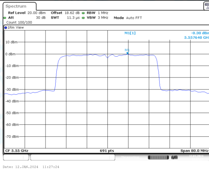
11AX40-CDD_Ant2_5550
