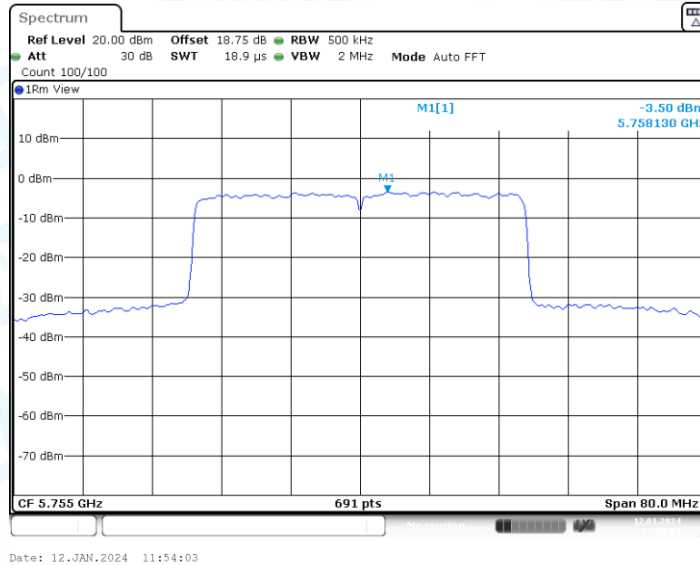
11AX40-CDD_Ant2_5755
