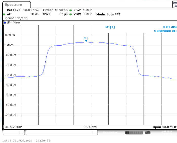
11AX20-CDD_Ant2_5700
