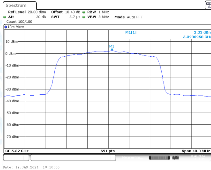
11AX20-CDD_Ant2_5320
