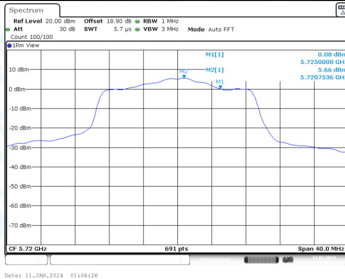
11AC20-CDD_Ant2_5720_UNII-2C
