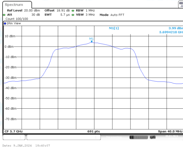
11AC20-CDD_Ant1_5720_UNII-2C
