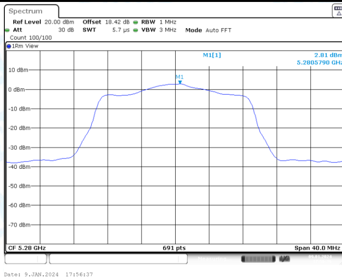
11AC20-CDD_Ant2_5280
