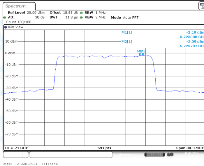
11AX40-CDD_Ant1_5710_UNII-3
