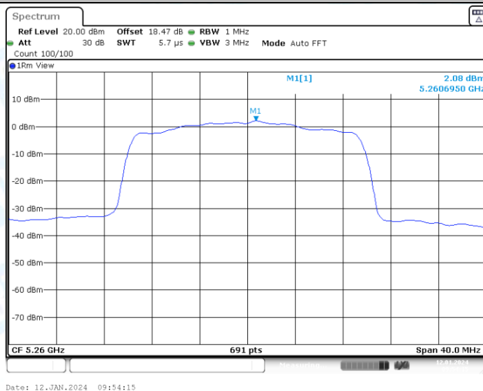
11AX20-CDD_Ant2_5260
