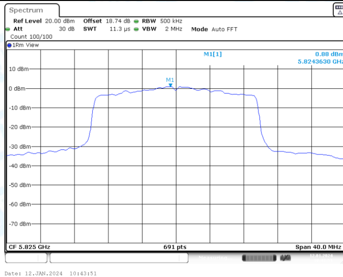
11AX20-CDD_Ant2_5825
