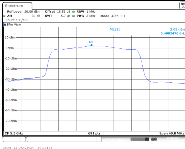
11AX20-CDD_Ant2_5500
