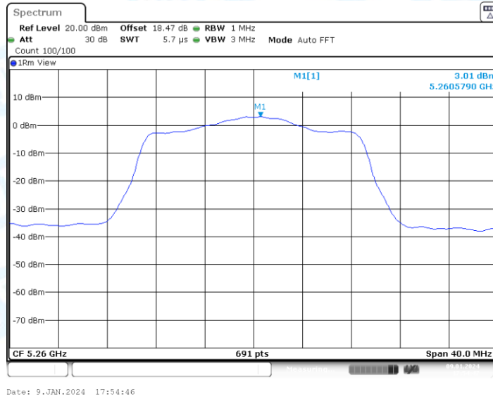
11AC20-CDD_Ant2_5260
