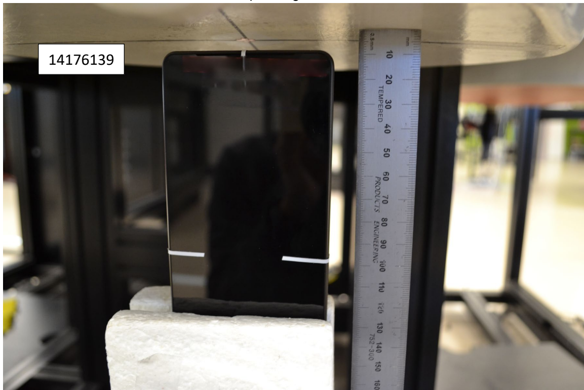
Hotspot, Edge 4, 10 mm
