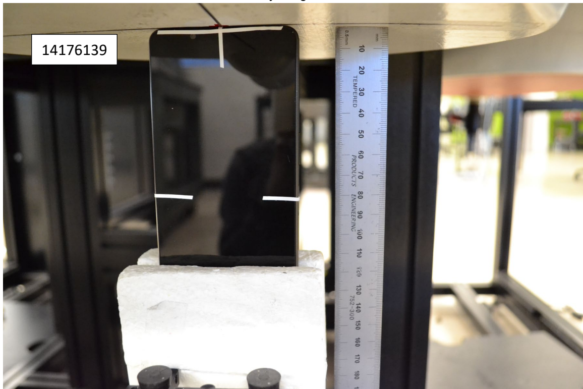
Extremity, Edge 2, 0 mm
