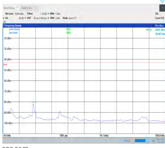
1-N66-PC3-15-40-H-1-DFT-PI2BPSK-Inner_1RB_L eft-1@1-0.009-0.15-Ant1-0.04--83.81--43-PASS
