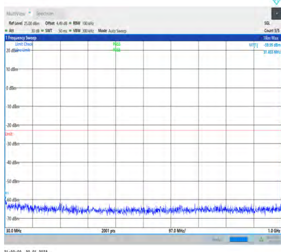
1-N66-PC3-15-40-H-1-DFT-PI2BPSK-Inner_1RB_L eft-1@1-30-1000-Ant1-31.46--59.99--23-PASS
