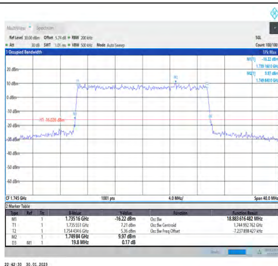
1-N66-PC3-15-20-M-7-CP-16QAM-Outer_Full-106@ 0-Ant1-18.884-19.800-≤20-PASS
