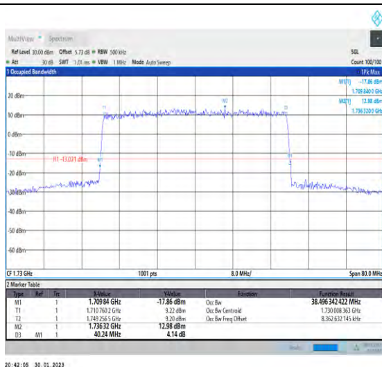
1-N66-PC3-15-40-L-1-DFT-QPSK-Outter_Full-216@ 0-Ant1-38.496-40.240-≤40-PASS
