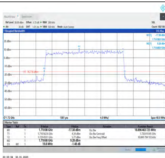
1-N66-PC3-15-20-L-8-CP-64QAM-Outer_Full-106@ 0-Ant1-18.896-19.800-≤20-PASS
