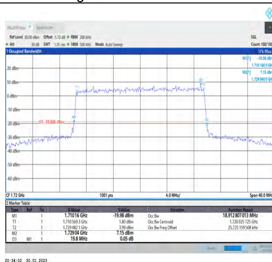
1-N66-PC3-15-20-L-9-CP-256QAM-Outer_Full-106 @0-Ant1-18.913-19.800-≤20-PASS
