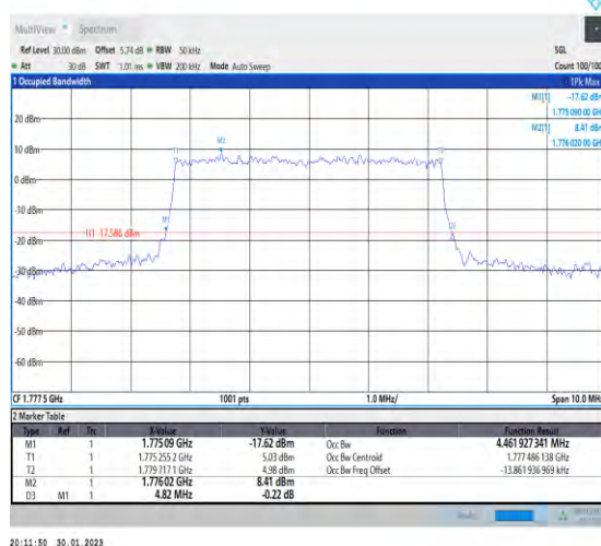
1-N66-PC3-15-5-H-6-CP-QPSK-Outer_Full-25@0-A nt1-4.462-4.820-≤5-PASS
