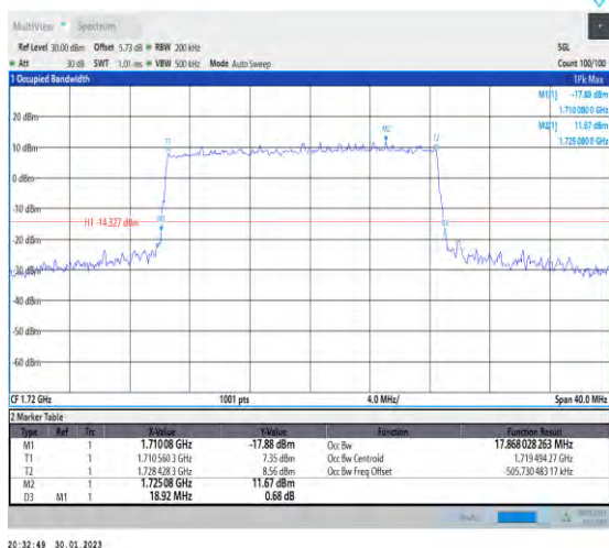
1-N66-PC3-15-20-L-4-DFT-64QAM-Outer_Full-100 @0-Ant1-17.868-18.920-≤20-PASS
