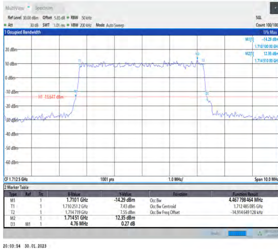
1-N66-PC3-15-5-L-1-DFT-QPSK-Outet_Full-25@0-A nt1-4.468-4.760-≤5-PASS
