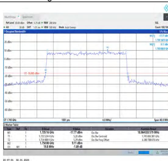
1-N66-PC3-15-20-M-8-CP-64QAM-Outer_Full-106@ 0-Ant1-18.964-19.800-≤20-PASS
