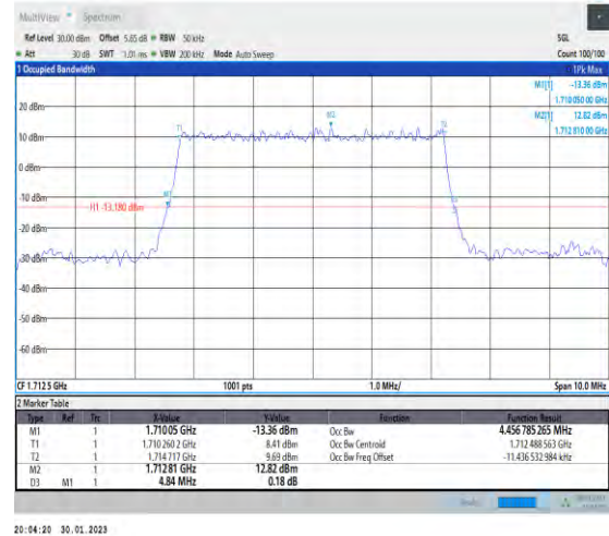
1-N66-PC3-15-5-L-2-DFT-PI2BPSK-Outet_Full-25@0-Ant1-4.457-4.840-≤5-PASS
