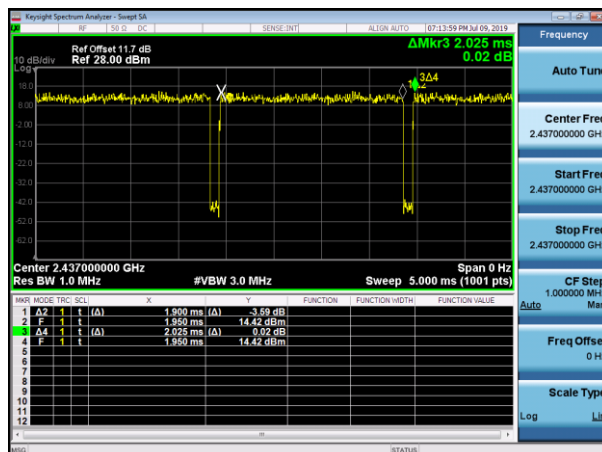
802.11n(20MHz)
