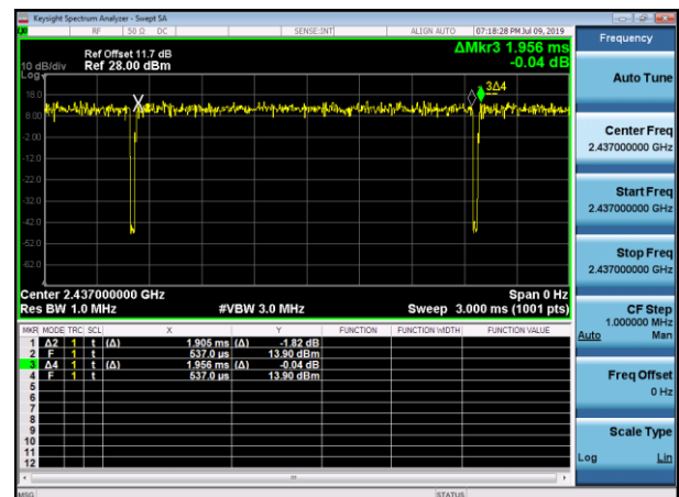
802.11ac(20MHz)
