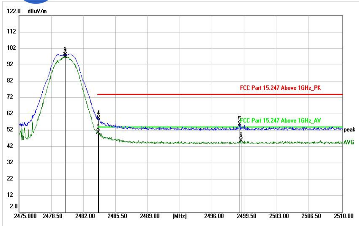
(LE 1M PHY_2480MHz, Antenna Horizontal)
