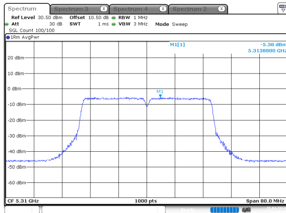
n40_5310MHz_Chain 2
