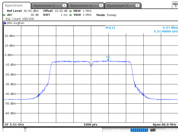
n40_5510MHz_Chain 2
