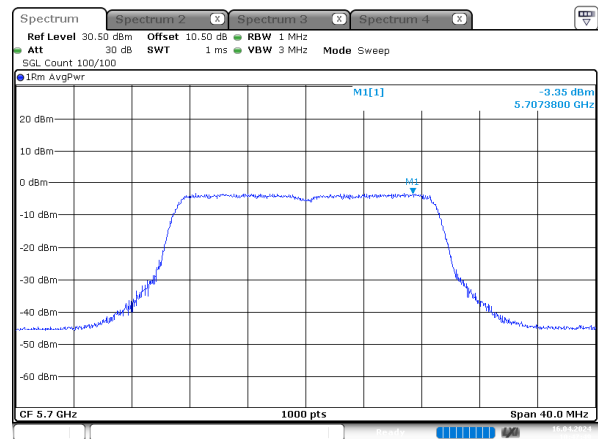
n20_5700MHz_Chain 3
