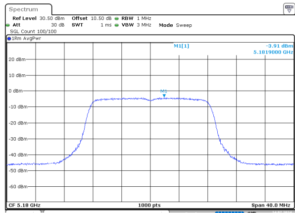
a_5180MHz_Chain 3
