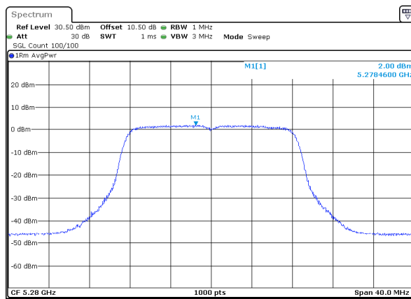
a_5280MHz_Chain 0
