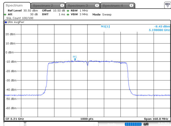
ac80_5210MHz_Chain 3
