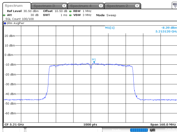
ac80_5210MHz_Chain 2
