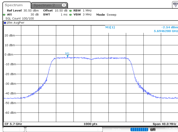
n20_5700MHz_Chain 0
