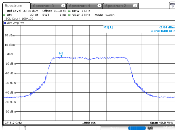
n20_5700MHz_Chain 2
