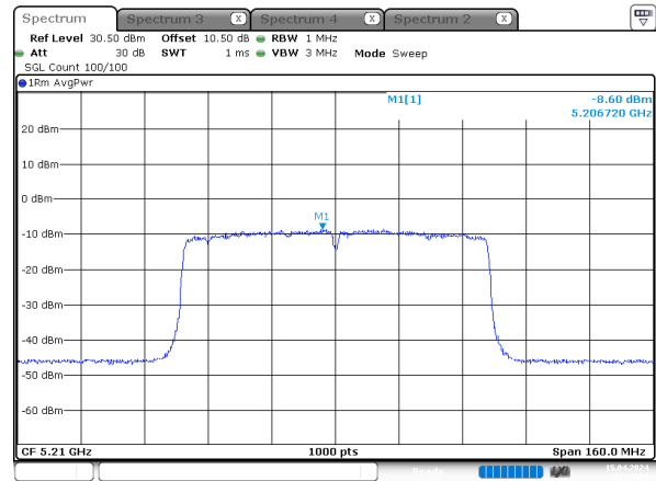
ac80_5210MHz_Chain 1
