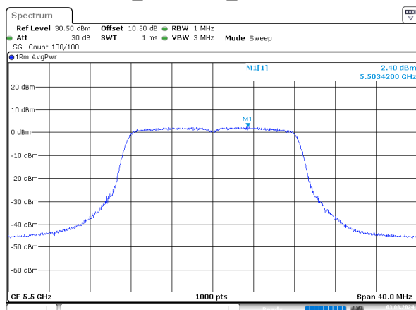
a_5500MHz_Chain 2
