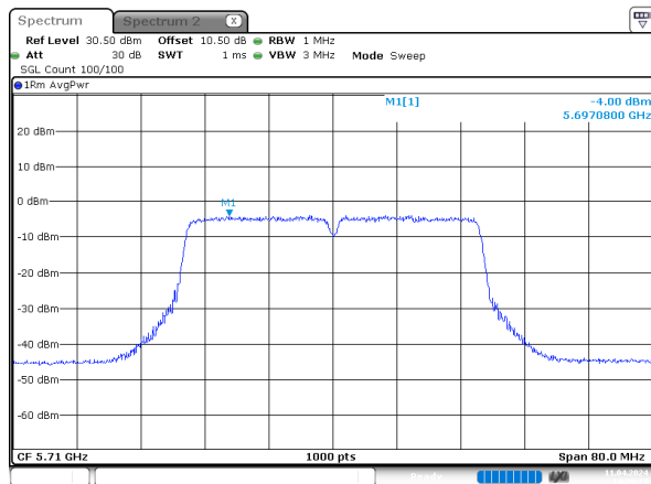
n40_5710MHz_Chain 0
