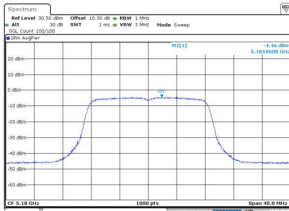
a_5180MHz_Chain 2
