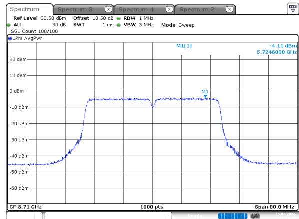
n40_5710MHz_Chain 1
