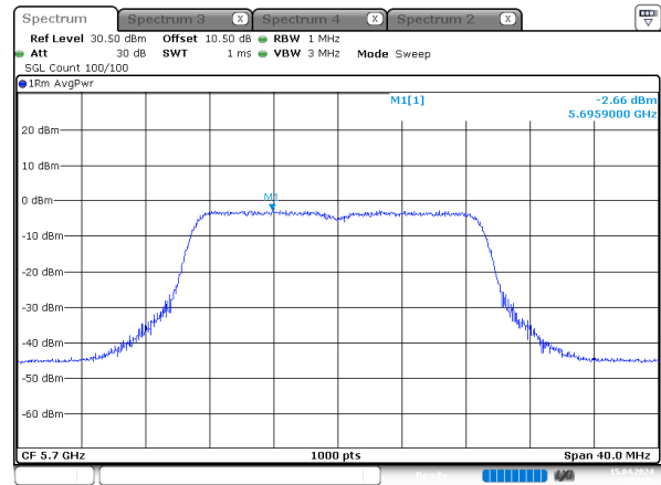
n20_5700MHz_Chain 1
