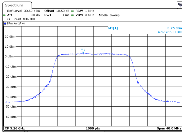
a_5260MHz_Chain 2
