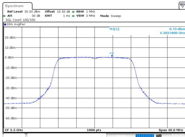
a_5500MHz_Chain 0
