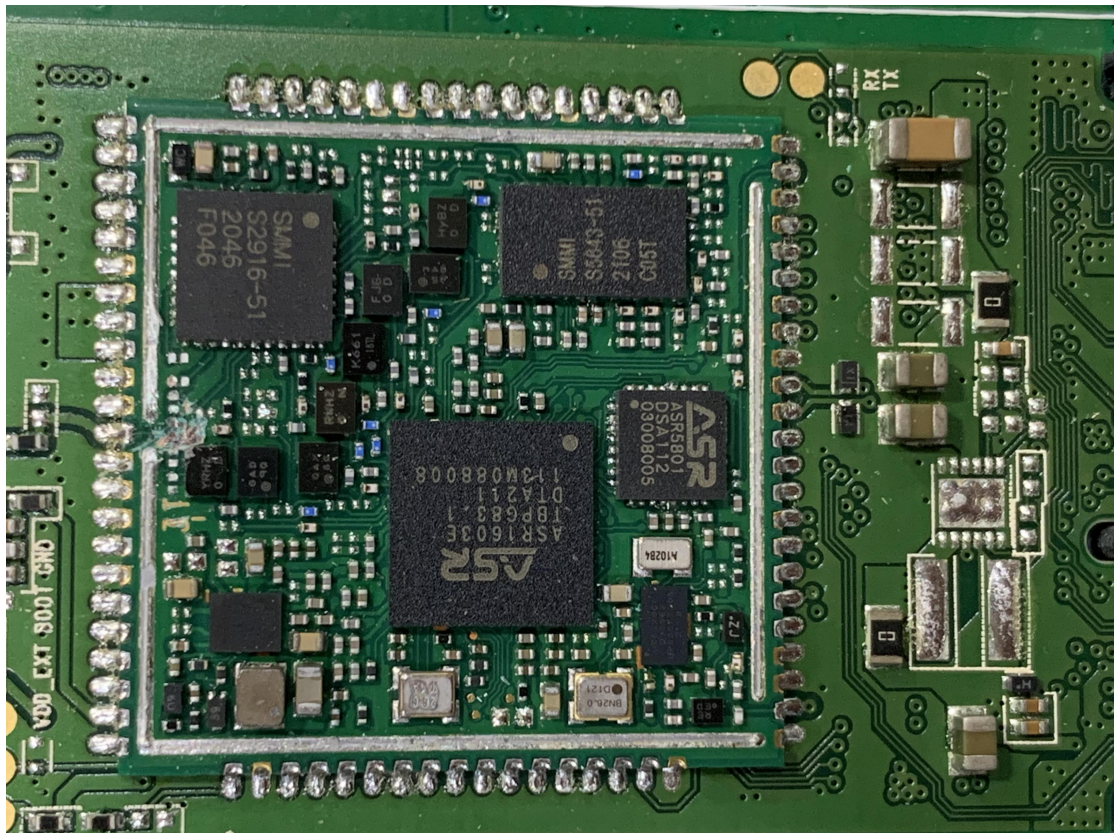
A7672SAminiPCIE
