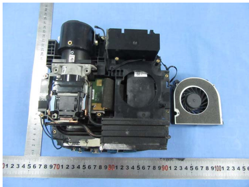
EUT – Cool Fan Uncovered View
