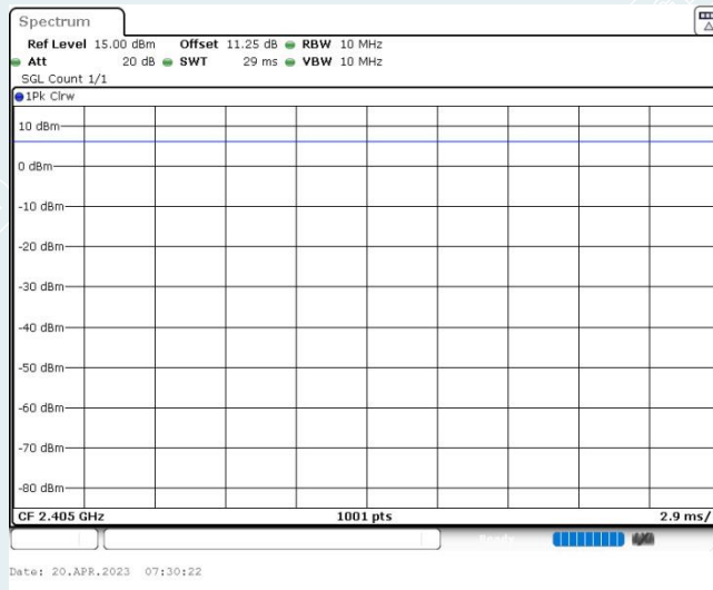
Lowest_2405MHz
