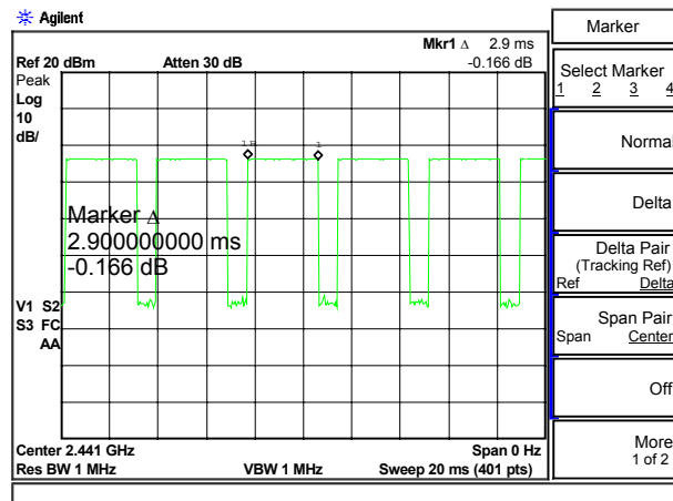
CH 39 2441MHz
