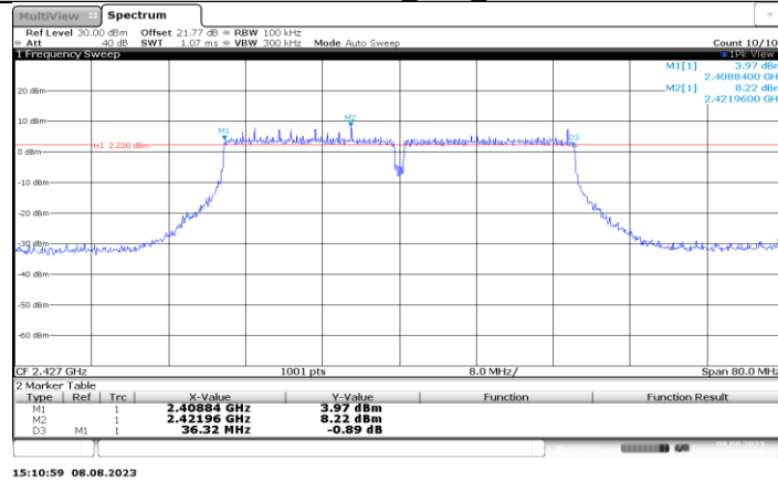
11N40MIMO_Ant4_2427
