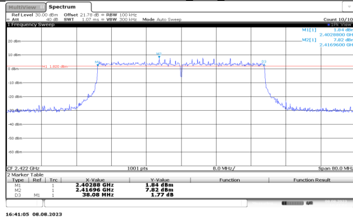
11BE40MIMO_Ant3_2422
