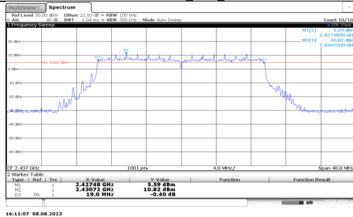
11BE20MIMO_Ant2_2437
