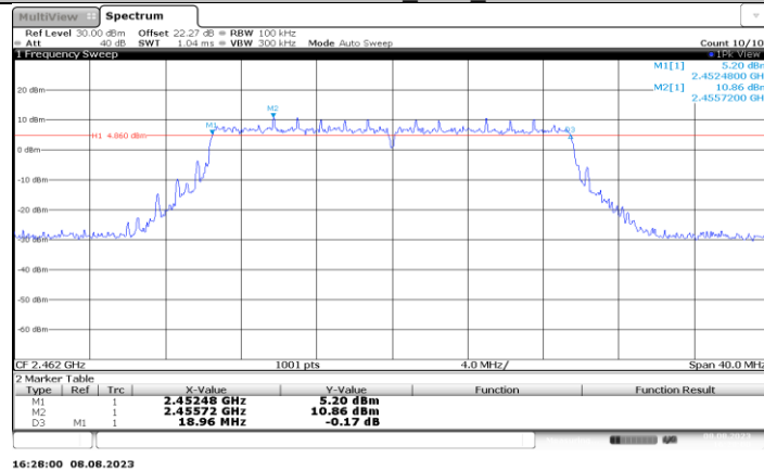
11BE20MIMO_Ant1_2462
