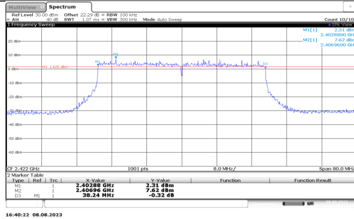
11BE40MIMO_Ant2_2422
