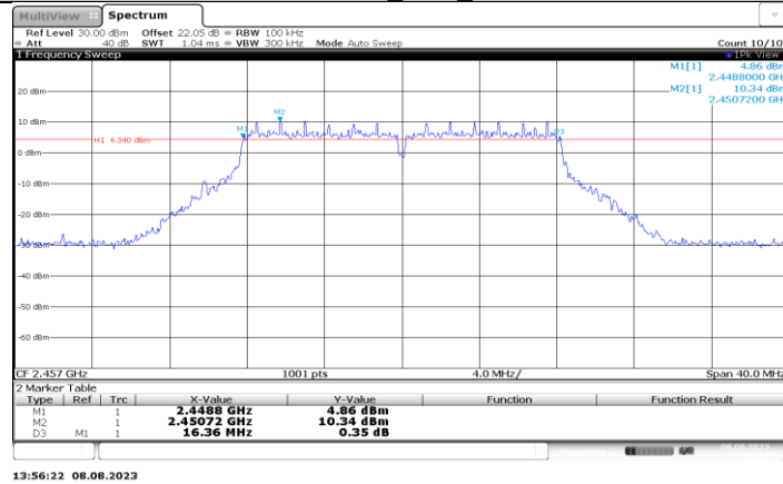
11G-CDD_Ant1_2457
