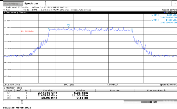
11BE20MIMO_Ant4_2457
