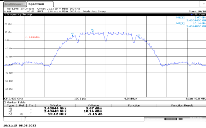
11B-CDD_Ant3_2437
