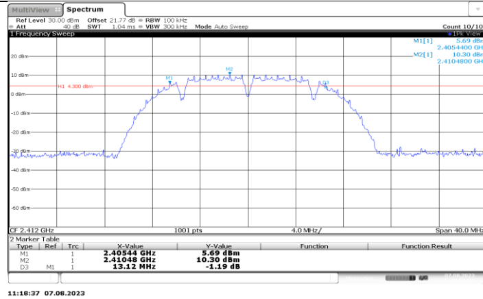
11B-CDD_Ant4_2412
