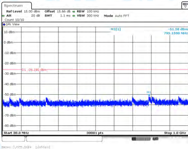
11G-Ant1-2412-30~1000-PASS
