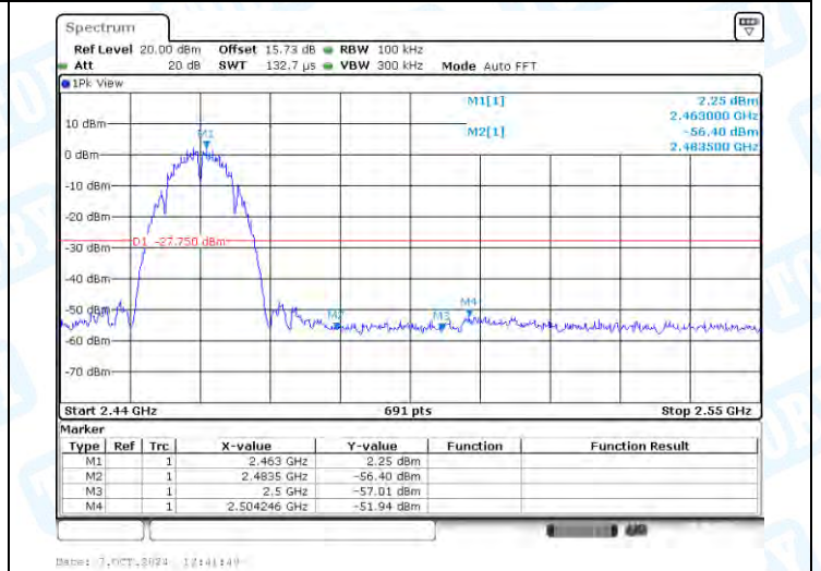
11B-Ant2-2462-PASS
