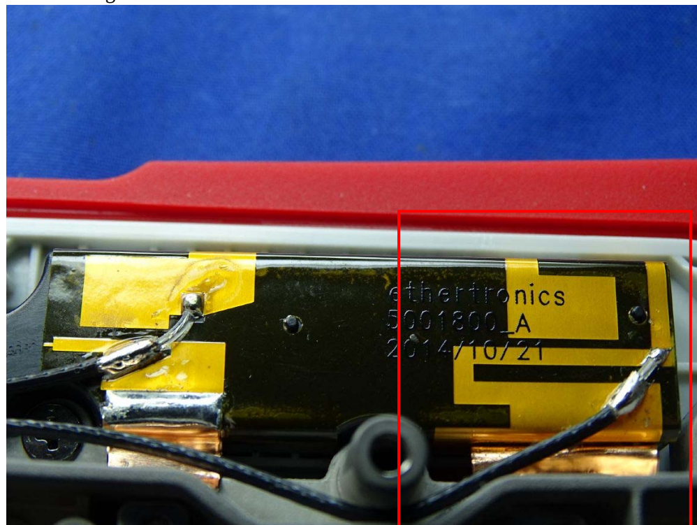
(40) EUT Photo - right WLAN Aux Ant
