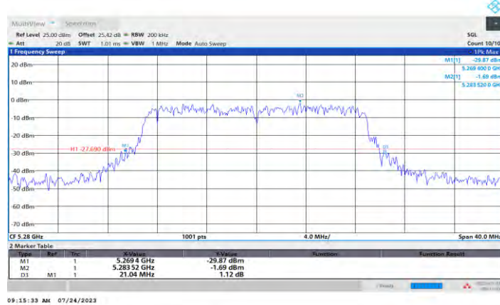
11N20SISO_Ant3_5280
