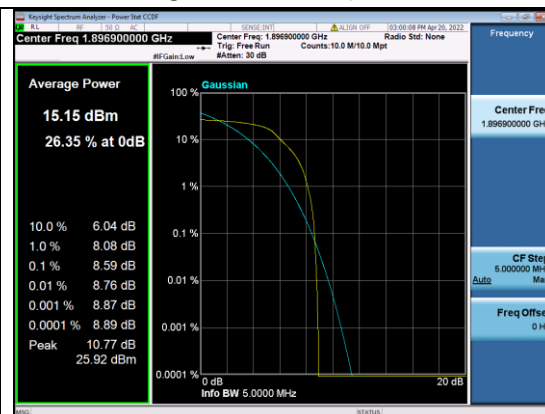
B25-20M-High CH-PAPR-QPSK
