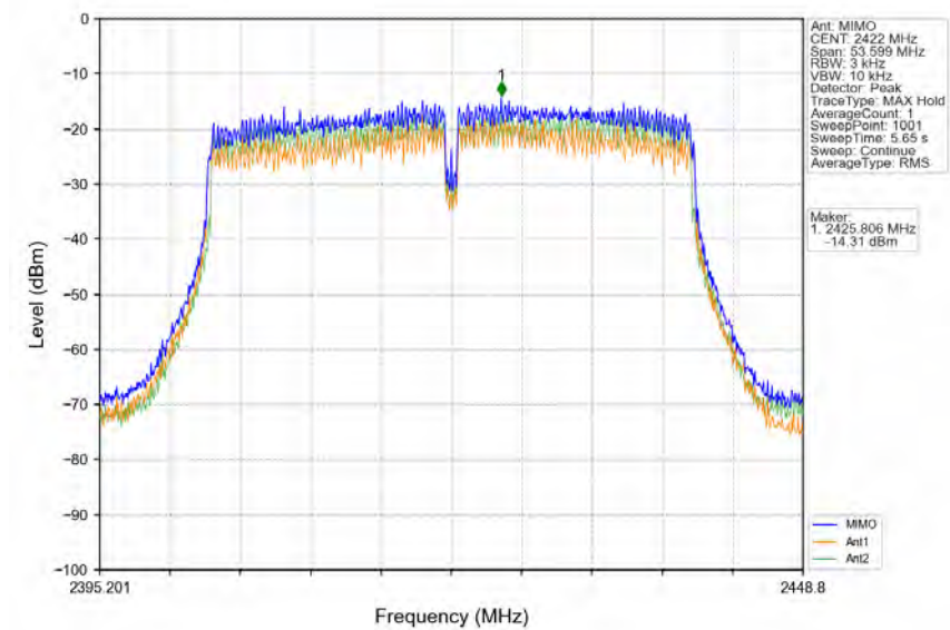
802.11n(HT40) LCH 2422MHz MIMO NTV
