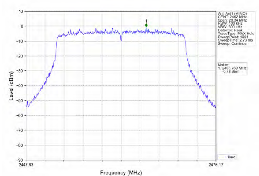
802.11ax(HEW20) HCH 2462MHz RU242 Left Ant1 (MIMO) NTN
