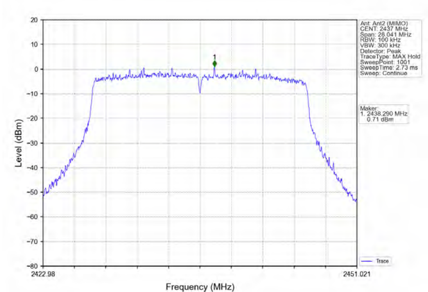
802.11ax(HEW20) MCH 2437MHz RU242 Left Ant2 (MIMO) NTVN
