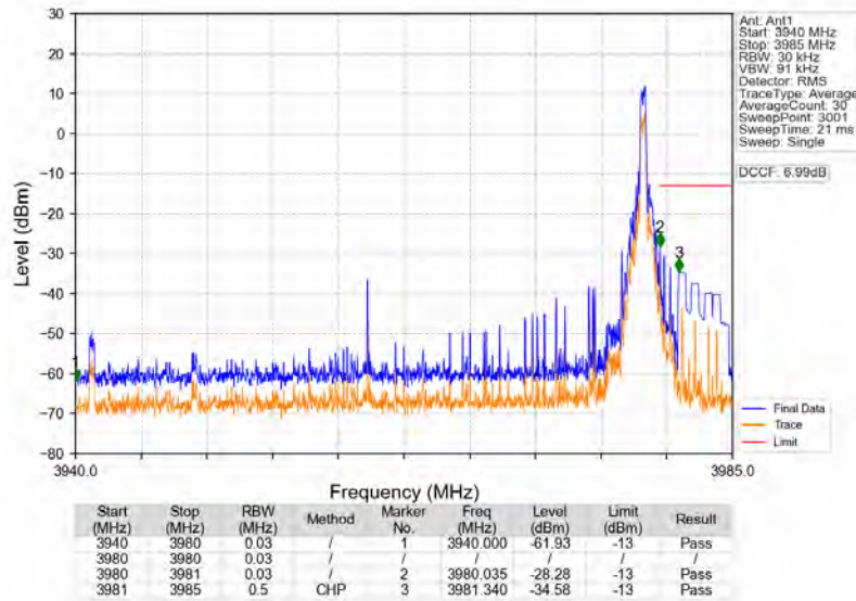
n77a 30kHz SISO NTN 40MHz CP-OFDM QPSK 3960MHz Edge 1RB Right
