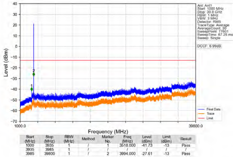
n77a 30kHz SISO NTN 40MHz DFT-s-OFDM QPSK 3960MHz Edge 1RB Right
