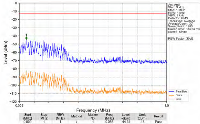
n77a 30kHz SISO NTN 40MHz CP-OFDM QPSK 3960MHz Edge 1RB Right
