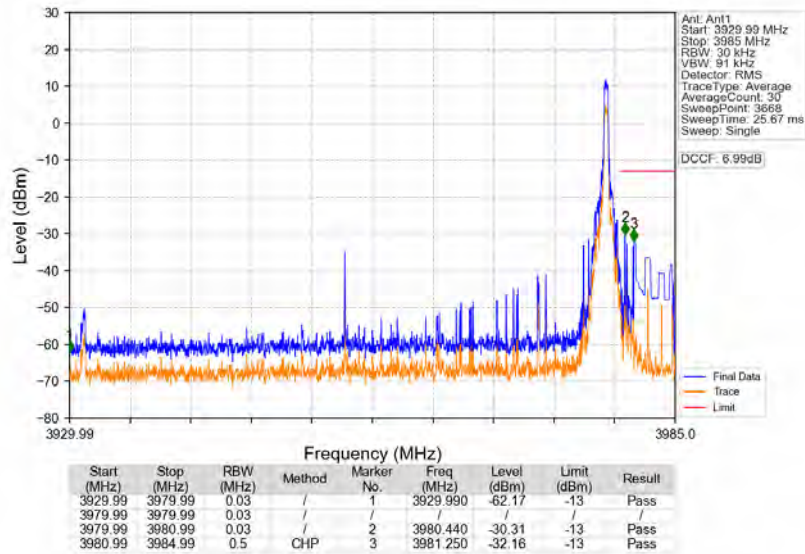
n77a 30kHz SISO NTN 50MHz CP-OFDM QPSK 3954.99MHz Edge 1RB Right
