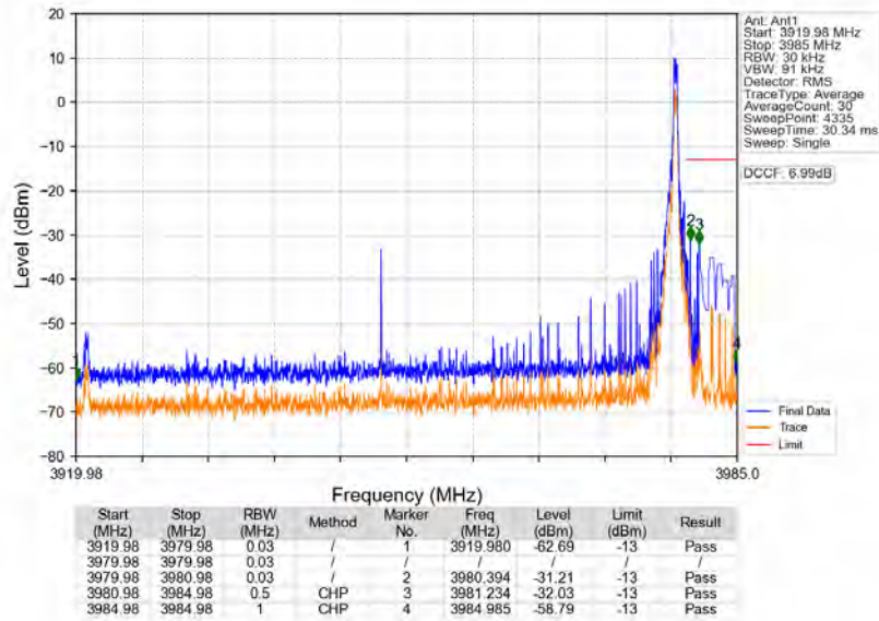
n77a 30kHz SISO NTN 60MHz CP-OFDM QPSK 3949.98MHz Edge 1RB Right
