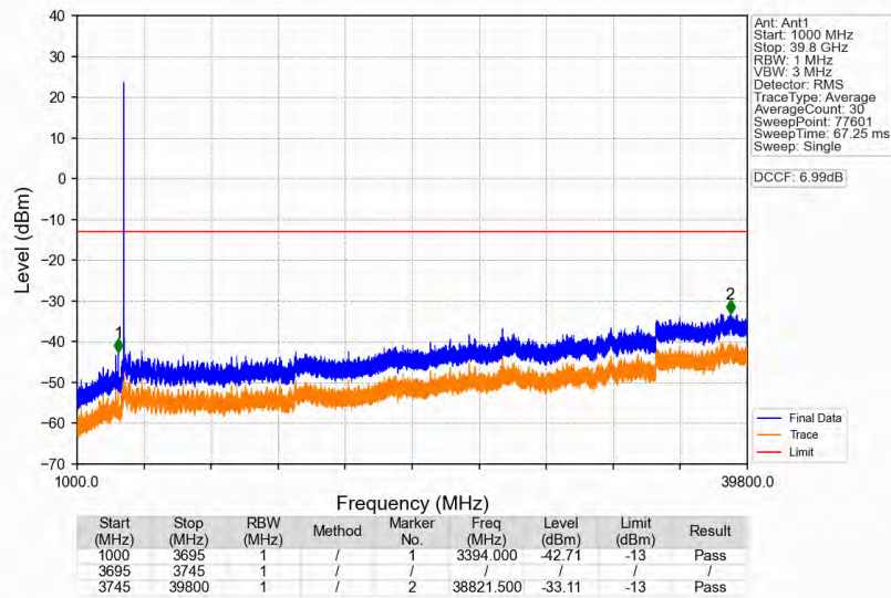
n77a 30kHz SISO NTN 40MHz DFT-s-OFDM PI/2 BPSK 3720MHz Edge 1RB Left
