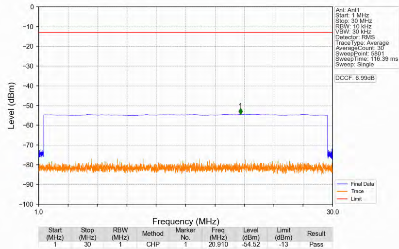
n77a 30kHz SISO NTN 40MHz DFT-s-OFDM QPSK 3960MHz Edge 1RB Right
