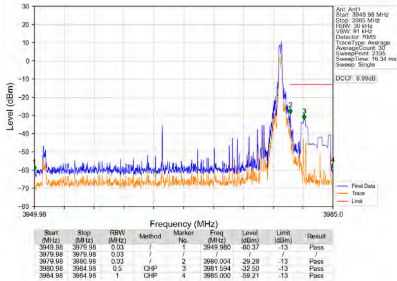
n77a 30kHz SISO NTN 30MHz CP-OFDM QPSK 3964.98MHz Edge 1RB Right
