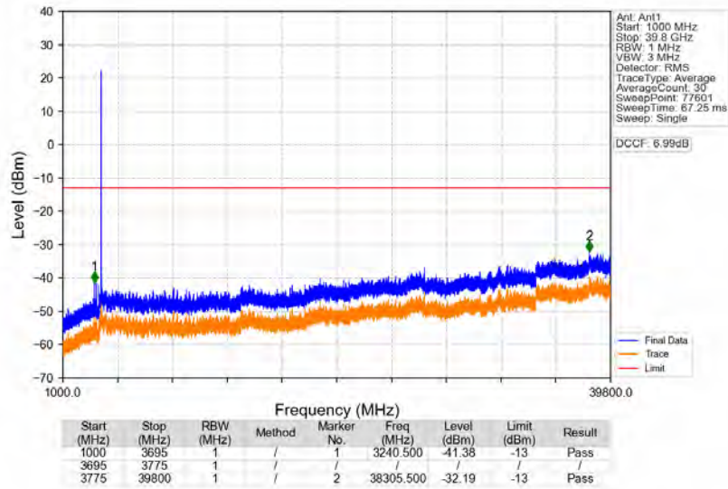
n77a 30kHz SISO NTN 70MHz DFT-s-OFDM PI/2 BPSK 3735MHz Edge 1RB Left
