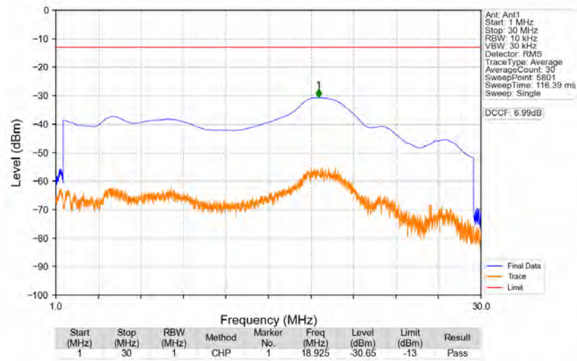
n77a 30kHz SISO NTN 30MHz CP-OFDM QPSK 3964.98MHz Edge 1RB Right
