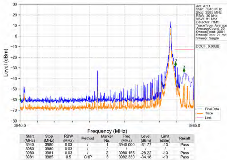
n77a 30kHz SISO NTN 40MHz DFT-s-OFDM QPSK 3960MHz Edge 1RB Right
