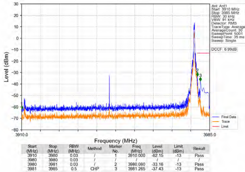
n77a 30kHz SISO NTN 70MHz DFT-s-OFDM QPSK 3945MHz Edge 1RB Right
