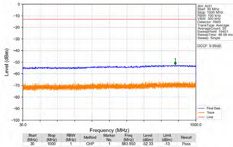
n77a 30kHz SISO NTN 70MHz DFT-s-OFDM QPSK 3945MHz Edge 1RB Right
