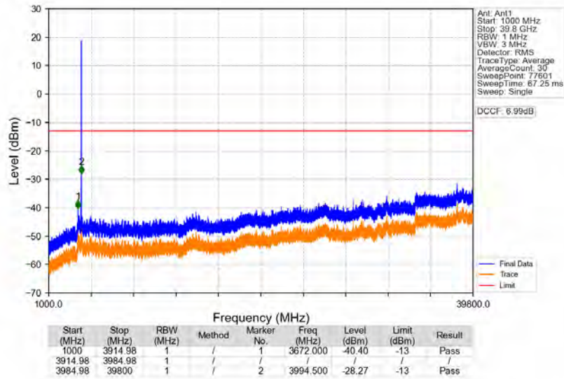
n77a 30kHz SISO NTN 60MHz CP-OFDM QPSK 3949.98MHz Edge 1RB Right
