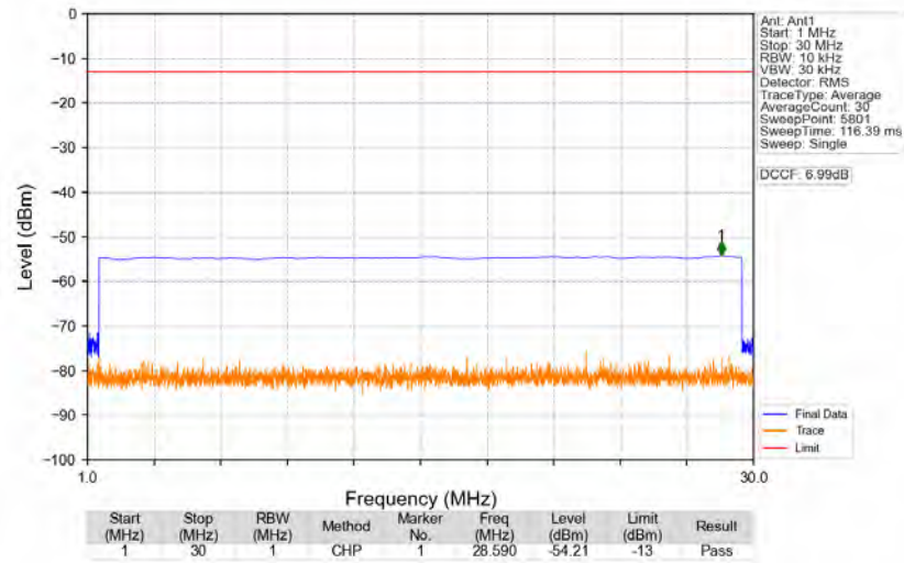
n77a 30kHz SISO NTN 60MHz CP-OFDM QPSK 3949.98MHz Edge 1RB Right
