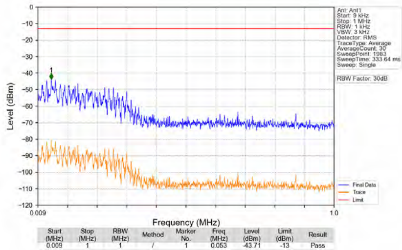
n77a 30kHz SISO NTN 50MHz CP-OFDM QPSK 3954.99MHz Edge 1RB Right
