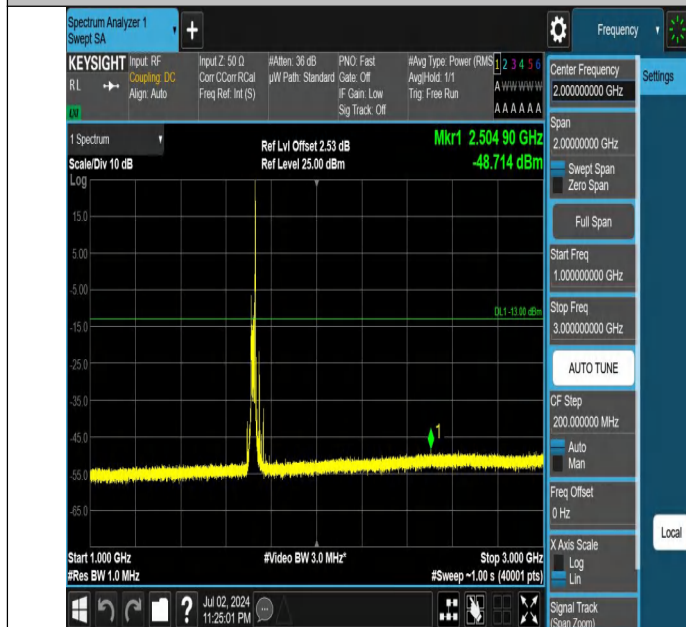
Band66-20MHz-QPSK-132072-1RB#99-1000~3000-PASS
