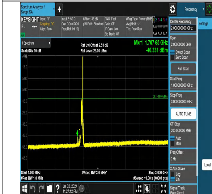
Band66-20MHz-QPSK-132572-1RB#99-1000~3000-PASS
