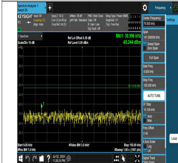
Band66-20MHz-QPSK-132572-1RB#0-0.009~0.15-PASS
