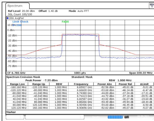
802.11ax (80MHz) 6785MHz Chain A NSS-4
