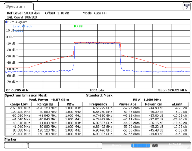
802.11ax (80MHz) 6785MHz Chain D NSS-4
