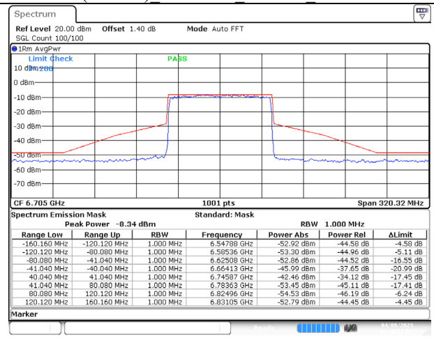
802.11ax (80MHz) 6705MHz Chain D NSS-4
