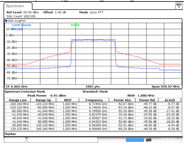
802.11ax (80MHz) 6865MHz Chain B NSS-4
