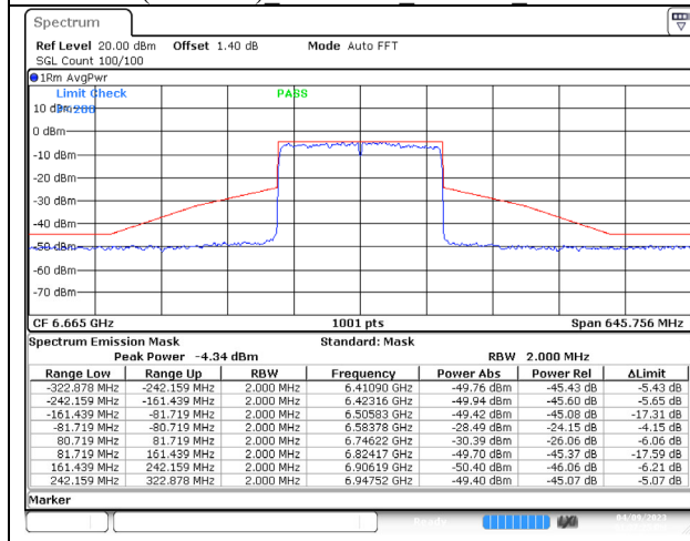
802.11ax (160MHz) 6665MHz Chain A NSS-4
