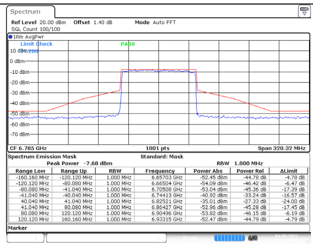
802.11ax (80MHz) 6785MHz Chain B NSS-4
