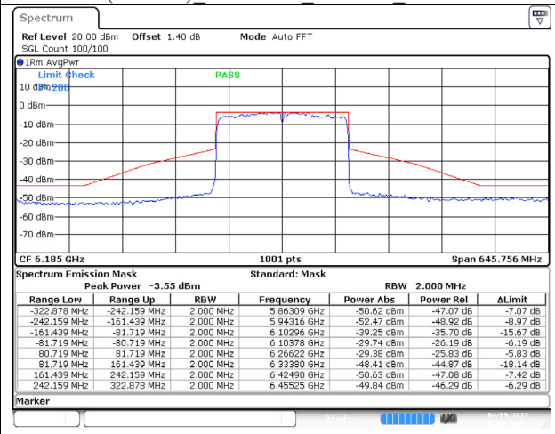
802.11ax (160MHz) 6185MHz Chain B NSS-4
