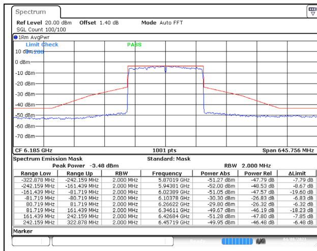
802.11ax (160MHz) 6185MHz Chain C NSS-4
