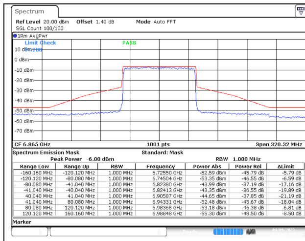
802.11ax (80MHz) 6865MHz Chain C NSS-4
