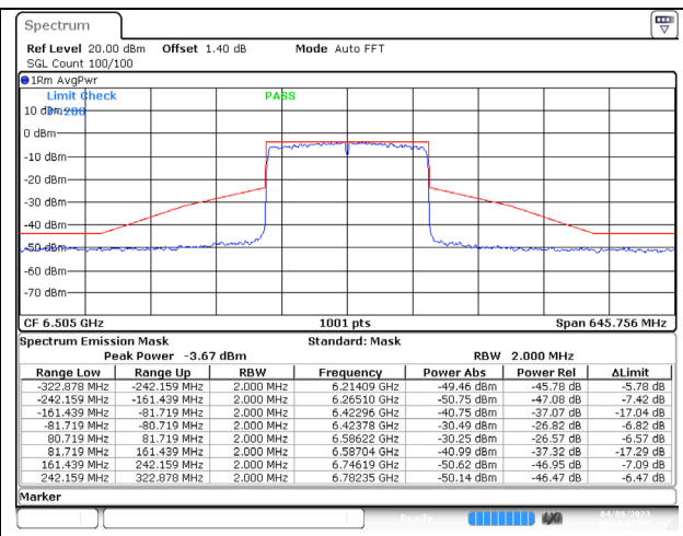
802.11ax (160MHz) 6505MHz Chain B NSS-4
