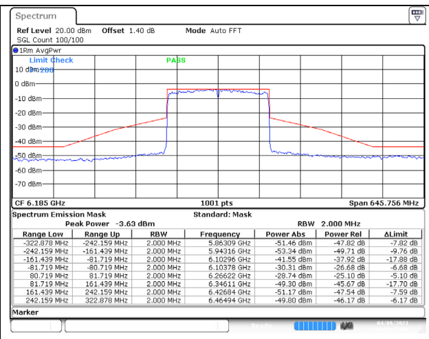
802.11ax (160MHz) 6185MHz Chain D NSS-4
