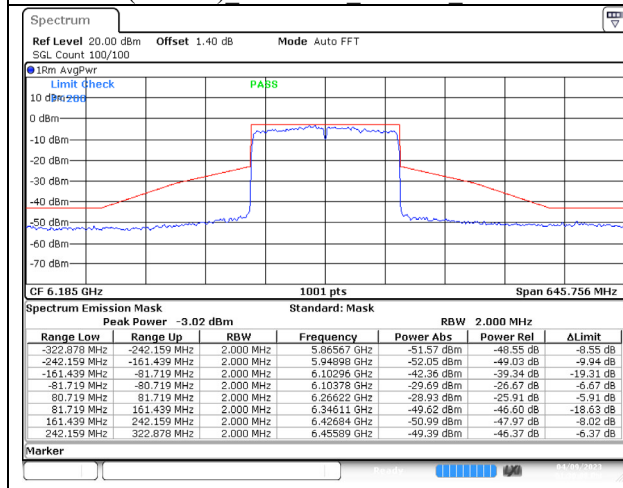
802.11ax (160MHz) 6185MHz Chain A NSS-4
