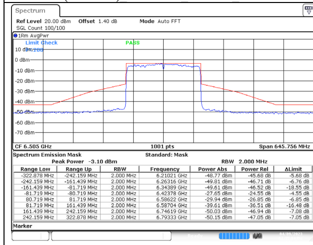
802.11ax (160MHz) 6505MHz Chain C NSS-4
