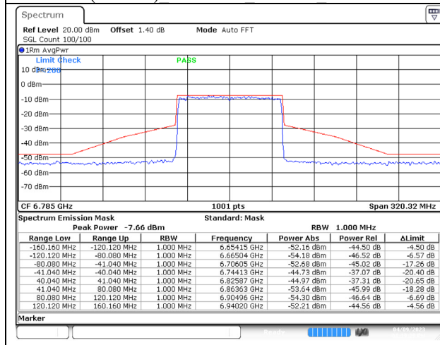
802.11ax (80MHz) 6785MHz Chain C NSS-4
