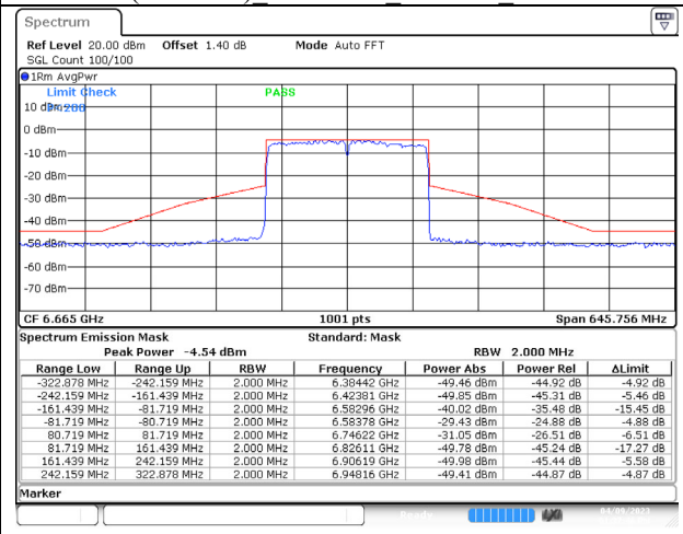
802.11ax (160MHz) 6665MHz Chain B NSS-4
