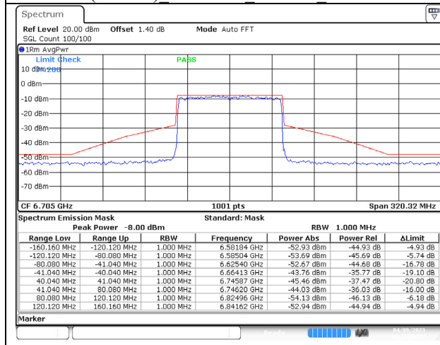
802.11ax (80MHz) 6705MHz Chain C NSS-4
