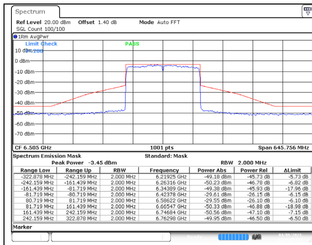
802.11ax (160MHz) 6505MHz Chain A NSS-4
