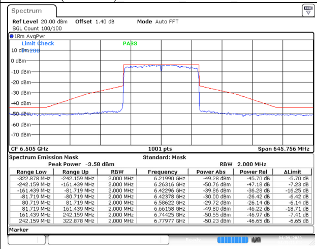
802.11ax (160MHz) 6505MHz Chain D NSS-4
