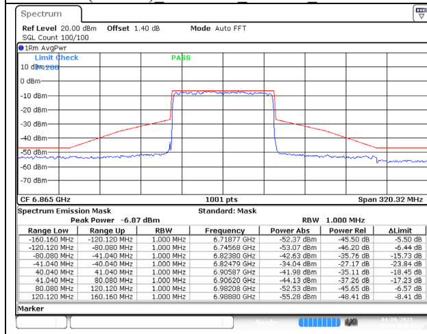
802.11ax (80MHz) 6865MHz Chain A NSS-4
