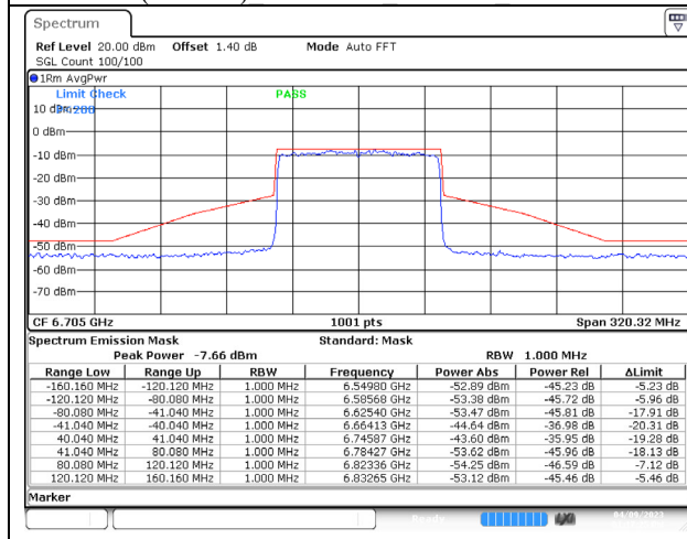
802.11ax (80MHz) 6705MHz Chain A NSS-4
