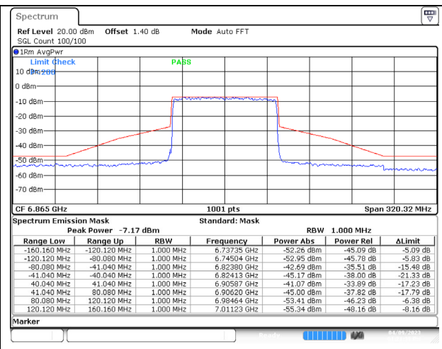
802.11ax (80MHz) 6865MHz Chain D NSS-4
