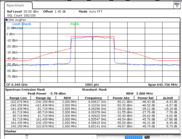
802.11ax (160MHz) 6345 CH79 4Tx Chain D NSS-4
