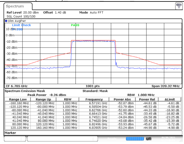
802.11ax (80MHz) 6705MHz Chain B NSS-4
