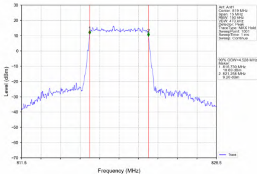
Band26a 5MHz QPSK MCH 819MHz RB 25 0 NTNV
