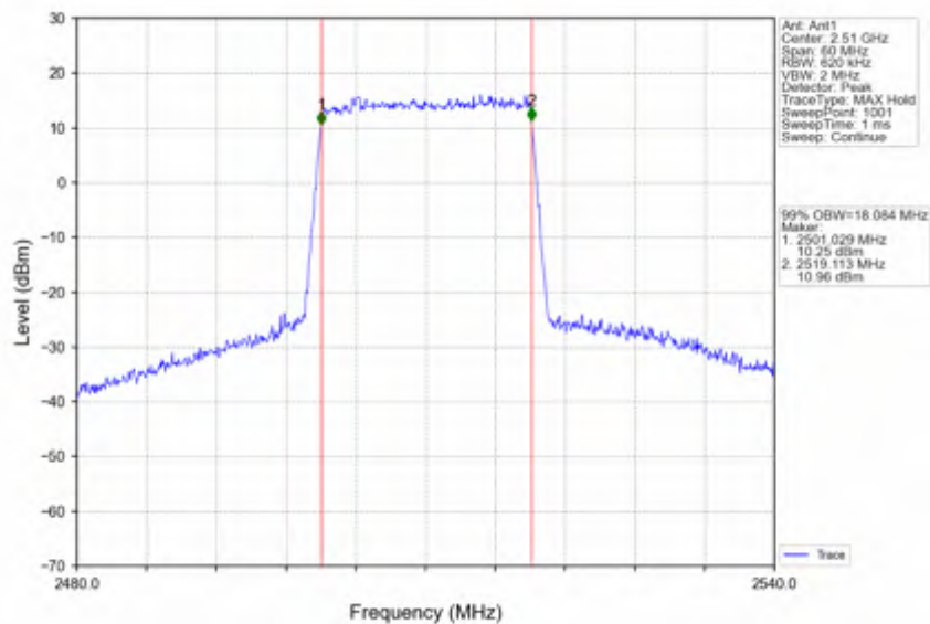
Band7_20MHz_256QAM_LCH_2510MHz_RB_100_0_NTNV
