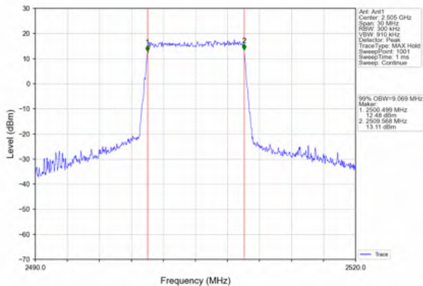
Band7 10MHz 16QAM LCH 2505MHz RB 50 0 NTNV
