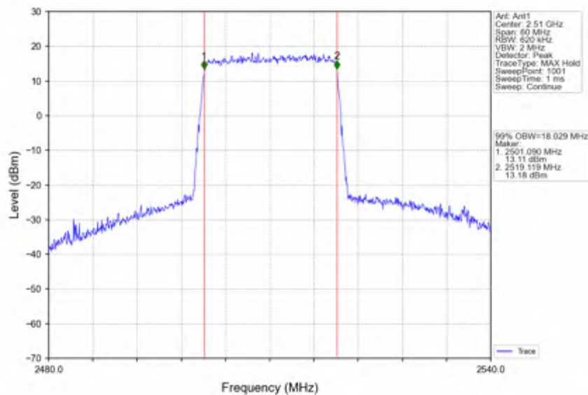
Band7 20MHz 16QAM LCH 2510MHz RB 100 0 NTNV
