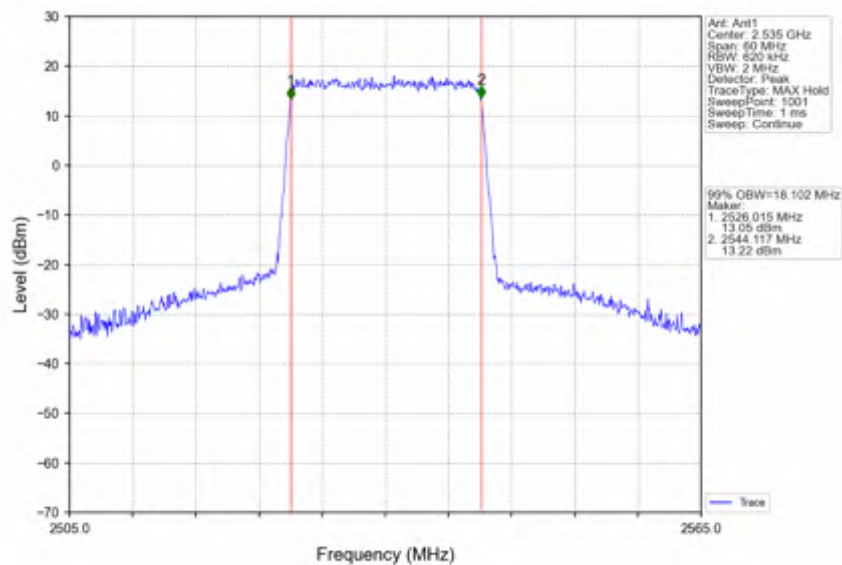
Band7_20MHz_64QAM_MCH_2535MHz_RB_100_0_NTNV
