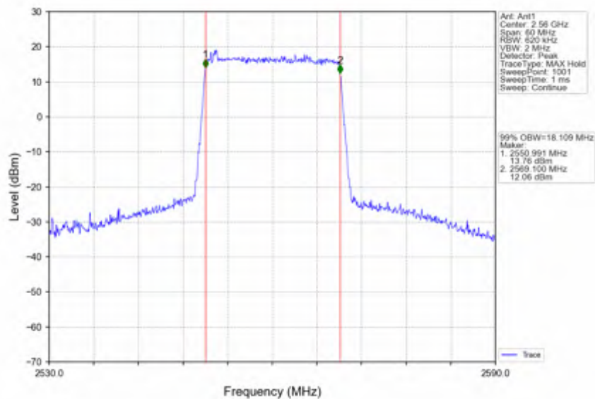
Band7_20MHz_16QAM_HCH_2560MHz_RB_100_0_NTNV
