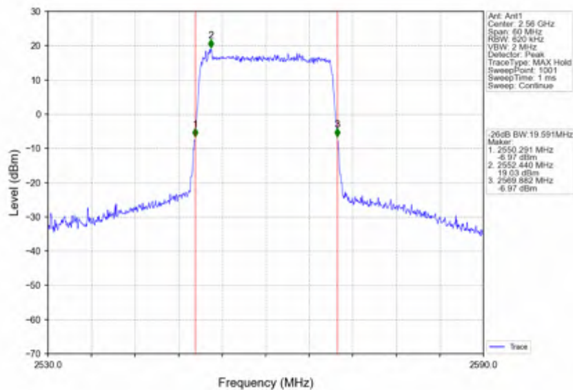
Band7_20MHz_16QAM_HCH_2560MHz_RB_100_0_NTNV
