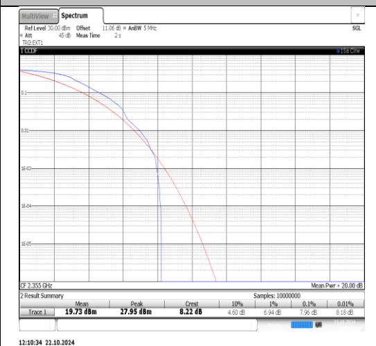
Band40(2350-2360)-10MHz-QPSK-39200-50RB#0-PASS
