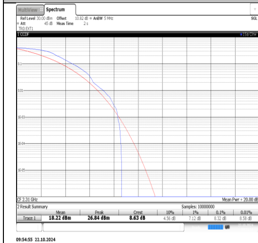
Band40(2305-2315)-10MHz-QPSK-38750-50RB#0-PASS
