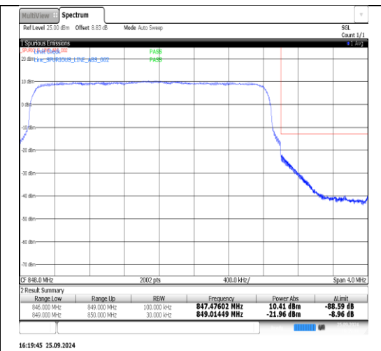
Band5-3MHz-QPSK-20635-1RB#14-PASS_Final1
