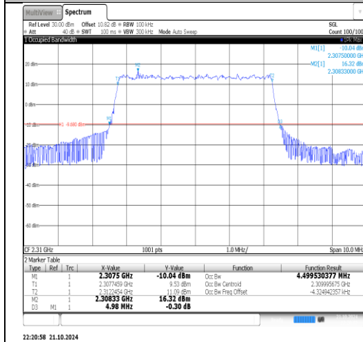
Band40(2305-2315)-10MHz-QPSK-38750- 50RB#0-PASS
