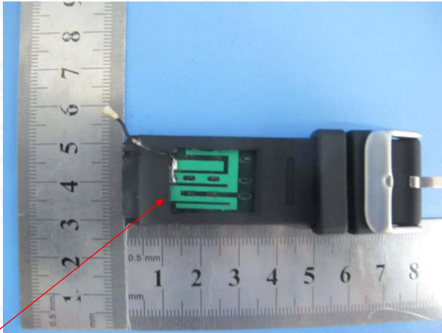
GSM&WCDMA Ant
