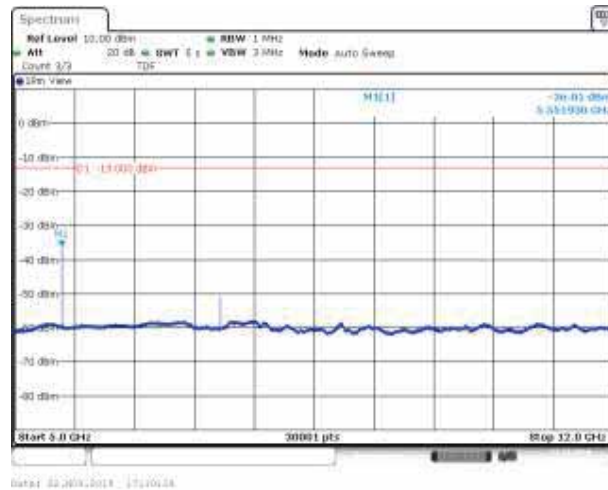
Band2_10MHz_QPSK_18650_1RB#0
