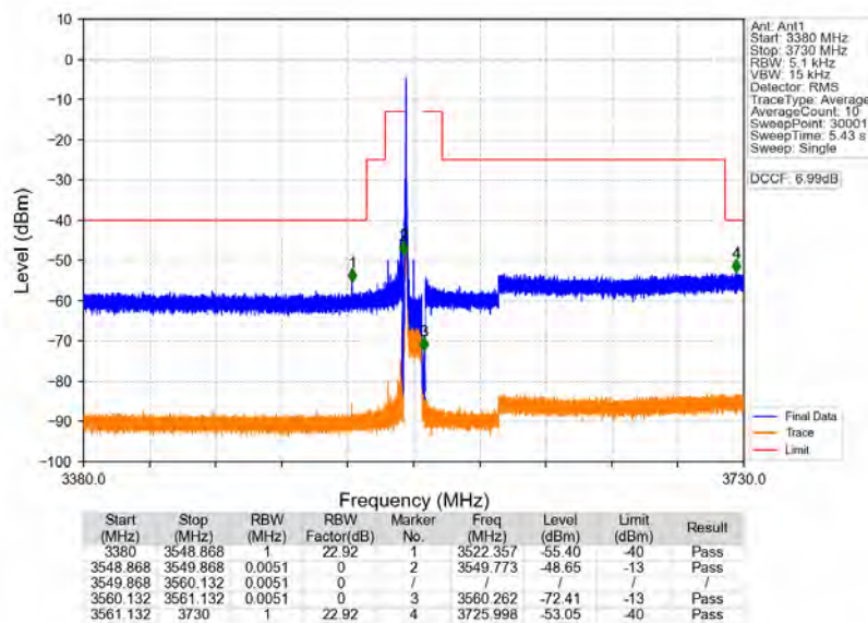
n78d 30kHz MIMO NTV 10MHz CP-OFDM QPSK 3555MHz Edge 1RB Left
