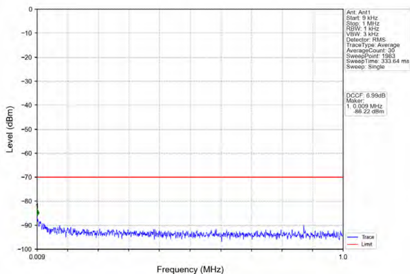
n78d 30kHz MIMO NTV 10MHz CP-OFDM QPSK 3555MHz Edge 1RB Left
